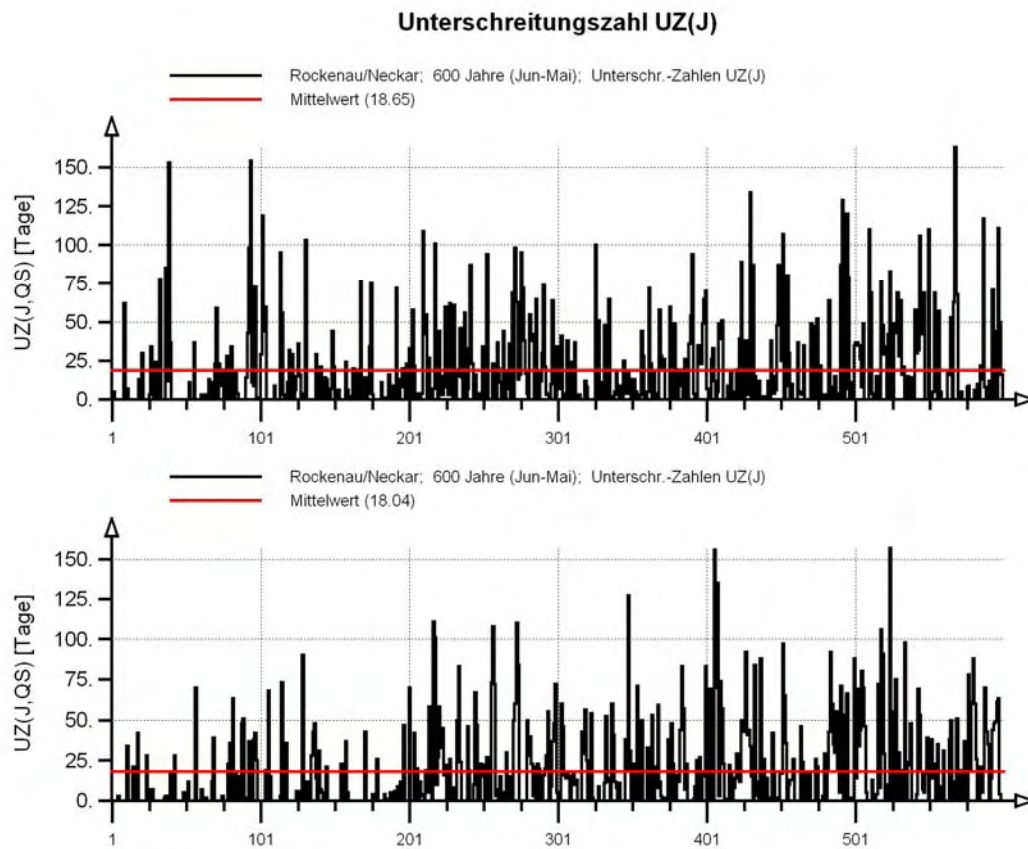
Abb. 2.4: Zeitreihe der jährlichen Unterschreitungszahl UZ(J) am Pegel Rockenau/Neckar abgeleitet aus den Abflusszeitreihen für den Ist-Zustand (oben) und den Zukunfts-Zustand (unten)
