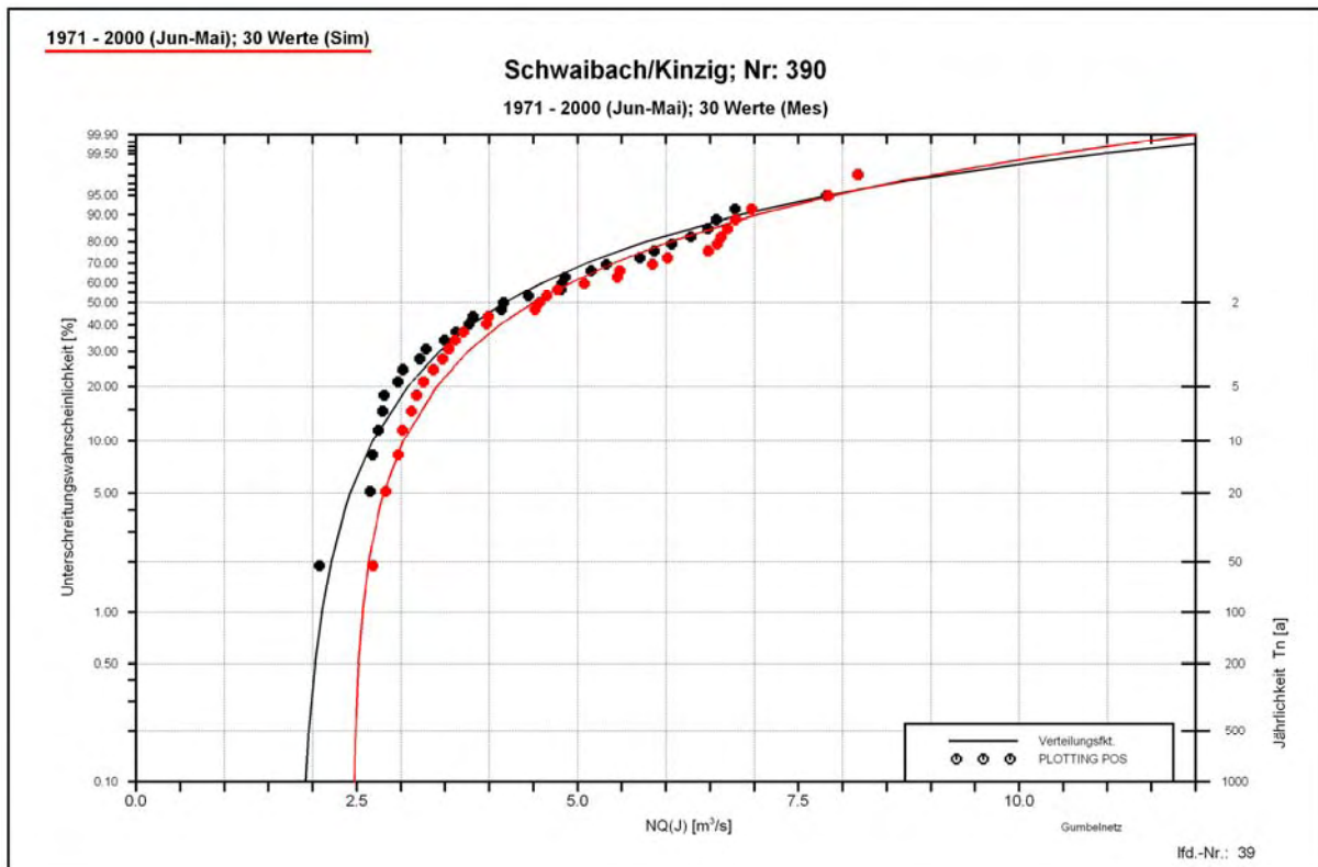
Abb. 5.1: Vergleich der Niedrigwasserstatistiken für die Niedrigwasserabflüsse des Jahres NQ(J), abgeleitet aus den Messwerten (schwarz) und den Abfluss-Simulationen (rot) am Pegel Schwaibach/Kinzig
