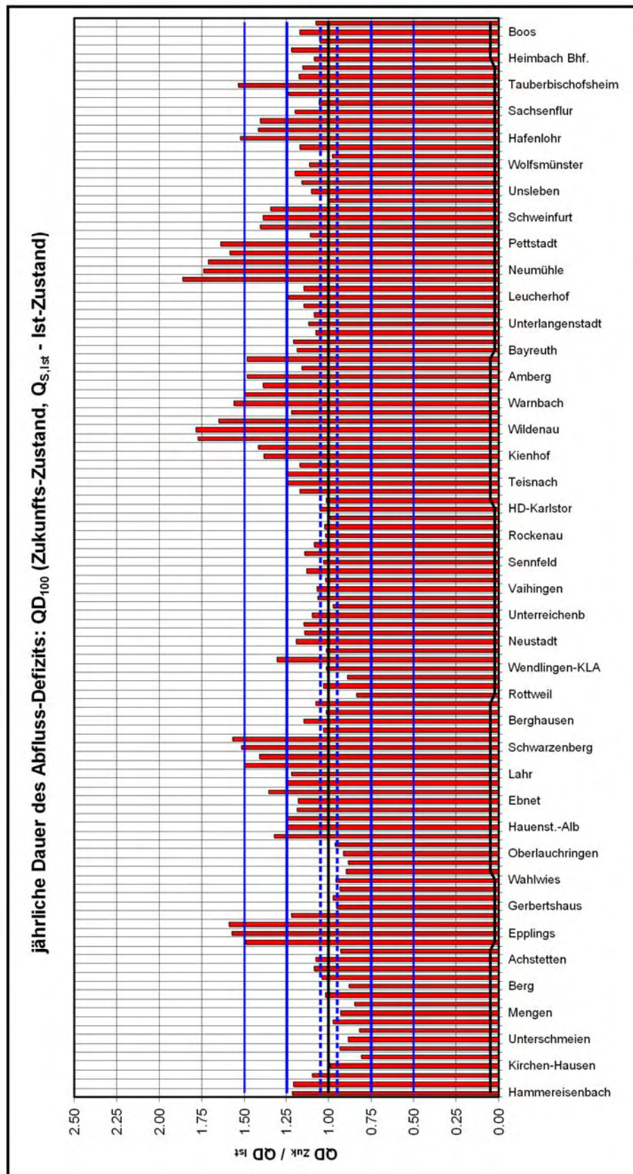
Abb. 6.11: Verhältnis der 100-jährlichen Dauer des Abflussdefizits QD_{100} aus dem Klimamodell für den Zukunfts-Zustand (2021 - 2050), bezogen auf den Schwellenwert MNQ_{ist} und dem Ist-Zustand (1971 - 2000) für alle einbezogenen Pegel und Gewässerstellen
