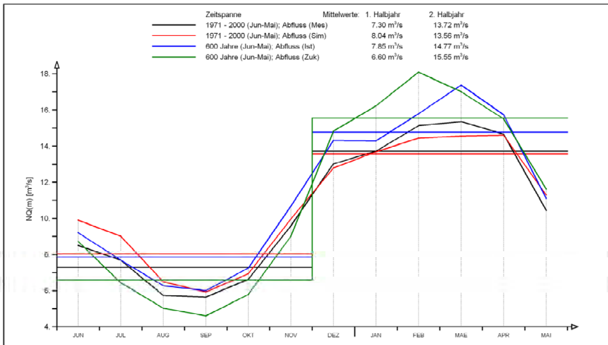
Abb. 4.1: Jahresgang der mittleren monatlichen Niedrigwasserabflüsse MNQ(m) am Pegel Schwaibach/Kinzig für die Messdaten (schwarz), die Abfluss-Simulation (rot) sowie Abflüsse auf Basis des Klimamodells für den Ist-Zustand (blau) und den Zukunfts-Zustand (grün) mit Jahresmittelwert (oberes Diagramm) und Halbjahresmittelwerten (unteres Diagramm)
