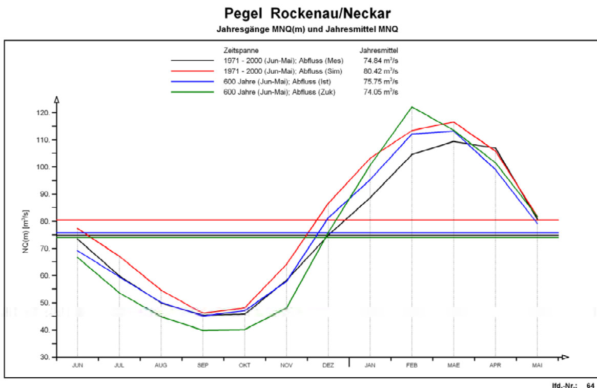
Abb. 3.1: Jahresgang der mittleren monatlichen Niedrigwasserabflüsse NQ(m) bezogen auf das hydrologische Jahr von Juni bis Mai und zugehörigem Jahresmittel MNQ am Pegel Rockenau/Neckar
