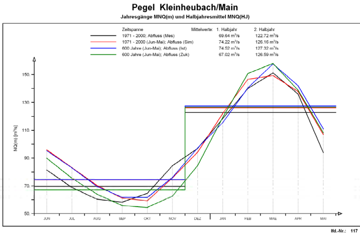
Abb. 4.2: Jahresgang der mittleren monatlichen Niedrigwasserabflüsse MNQ(m) am Pegel Kleinheubach/Main für die Messdaten (schwarz), die Abfluss-Simulation (rot) sowie Abflüsse auf Basis des Klimamodells für den Ist-Zustand (blau) und den Zukunfts-Zustand (grün) mit Jahresmittelwert (oberes Diagramm) und Halbjahresmittelwerten (unteres Diagramm)
