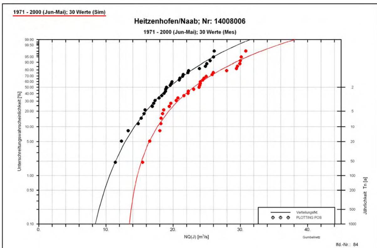
Abb. 5.2: Vergleich der Niedrigwasserstatistiken für die Niedrigwasserabflüsse des Jahres NQ(J), abgeleitet aus den Messwerten (schwarz) und den Abfluss-Simulationen (rot) am Pegel Heitzenhofen/Naab
