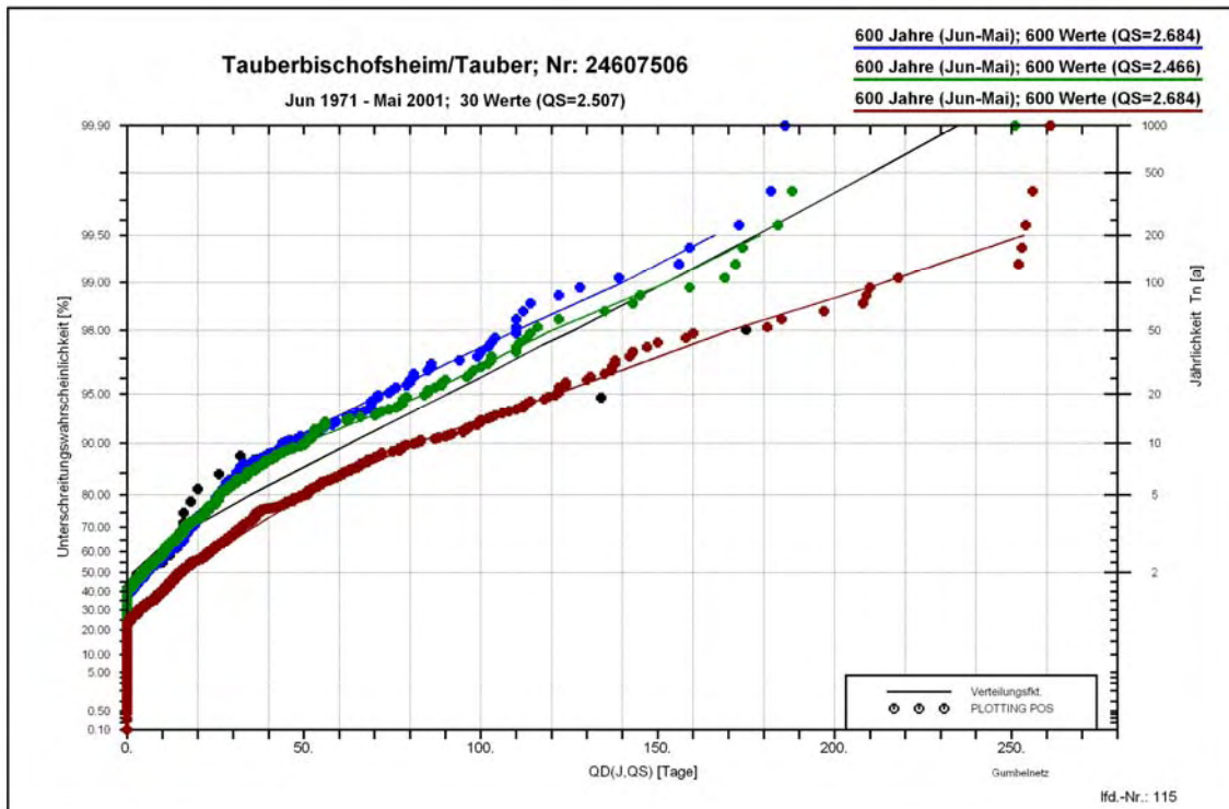
Abb. 6.5: Vergleich der Extremwertstatistiken für die jährliche Dauer des Abflussdefizits QD(J) , abgeleitet aus den Simulationen (schwarz) und den Berechnungen auf Basis des Klimamodells für den Ist-Zustand (blau) sowie für den Zukunfts-Zustand mit Q_S=MNQ_{Zuk} (grün) und Q_S=MNQ_{Ist} (braun) am Pegel Tauberbischofsheim-Tauber; Berechnungen mit dem Wasserhaushaltsmodell LARSIM (oben) und dem Modell ASGi/WaSiM-ETH (unten)
