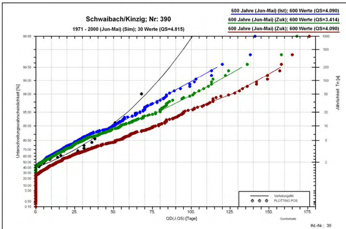
Abb. 6.1: Vergleich der Extremwertstatistiken für die jährliche Dauer des Abflussdefizits QD(J) , abgeleitet aus den Simulationen (schwarz) und den Berechnungen auf Basis des Klimamodells für den Ist-Zustand (blau) sowie für den Zukunfts-Zustand mit Q_S=MNQ_{Zuk} (grün) und Q_S=MNQ_{Ist} (braun) am Pegel Schwaibach/Kinzig
