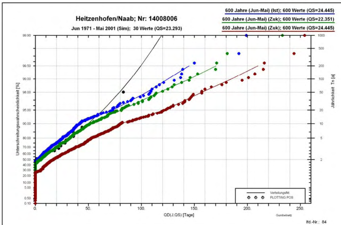
Abb. 6.2: Vergleich der Extremwertstatistiken für die jährliche Dauer des Abflussdefizits QD(J) , abgeleitet aus den Simulationen (schwarz) und den Berechnungen auf Basis des Klimamodells für den Ist-Zustand (blau) sowie für den Zukunfts-Zustand mit Q_S=MNQ_{Zuk} (grün) und Q_S=MNQ_{Ist} (braun) am Pegel Heitzenhofen/Naab
