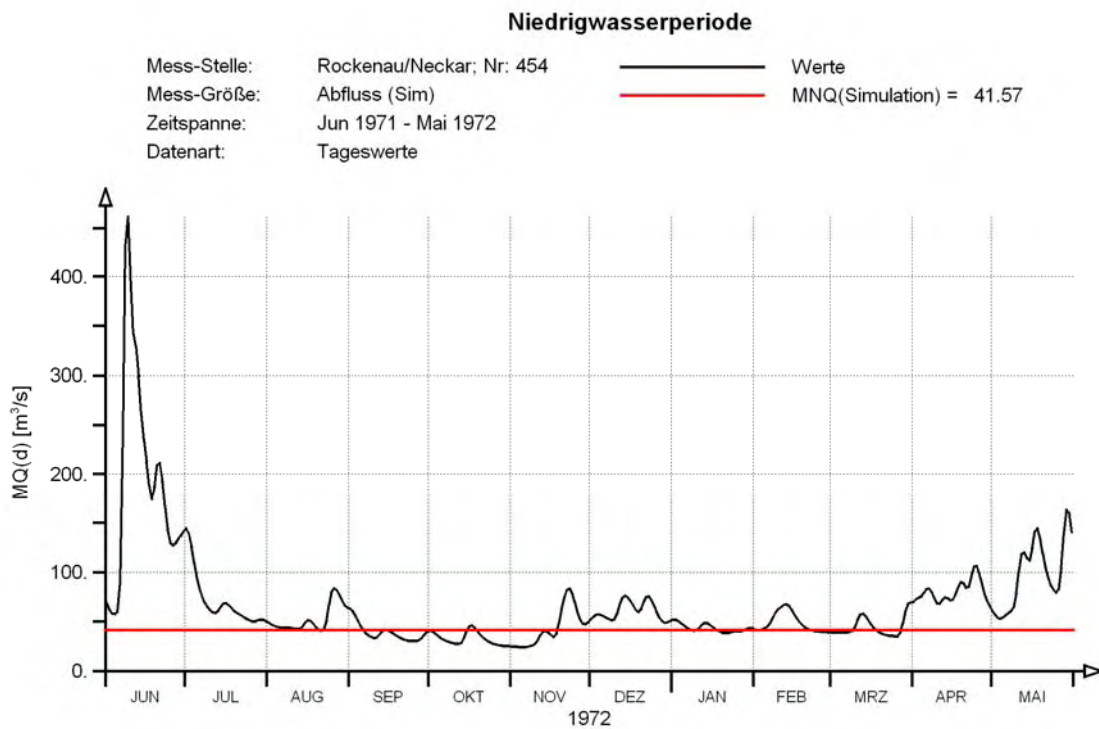
Abb. 2.3: Niedrigwasserperiode am Pegel Rockenau/Neckar für das hydrologische Jahr 1972 (Juni 1971 bis Mai 1972) mit mittlerem Niedrigwasserabfluss MNQ zur Definition der Kennwerte für Niedrigwasserperioden
