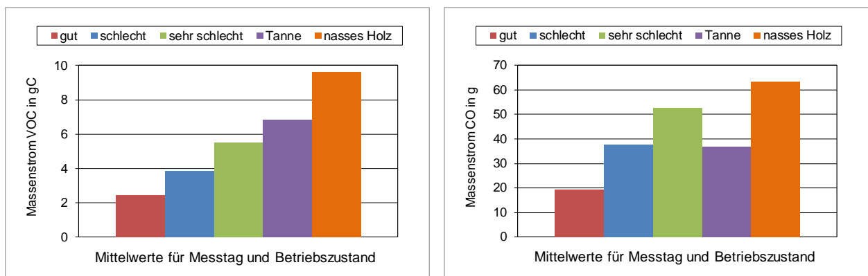
Abbildung 4.8 Mittelwerte (arithmetisch) der Massenströme für VOC und CO für alle Abbrände an einem Messtag (Anzünden und Abbrand von 3 Holzchargen) bei den verschiedenen Betriebszuständen gute, schlechte und sehr schlechte Verbrennung mit trockenem Buchenholz, gute Verbrennung mit Tannenholz und Verbrennung von nassem Buchenholz
