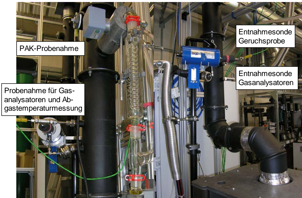
Abbildung 3.4 Schematischer Aufbau für PAK-Messungen (Bild oben) [Schlindwein, 2012] und Messstellen bei den Abbrandversuchen für die PAK-Bestimmung und die Geruchsprobe bei Messaufbau II (Bild unten)
