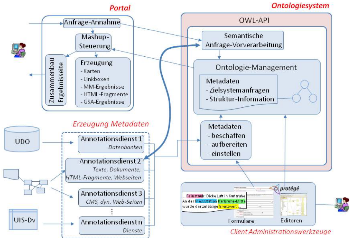
Abbildung 3: Erweiterte Architektur des Gesamtsystems
