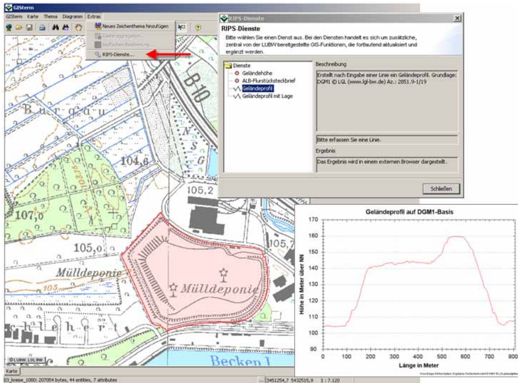
Abbildung 7: RIPS-Dienst, genutzt im GISterm zur Erstellung eines Deponieprofils
