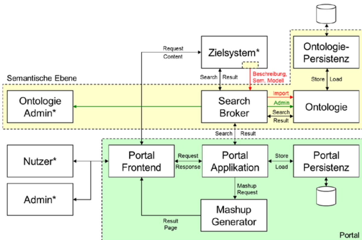
Abbildung 1: SUI-Architektur
