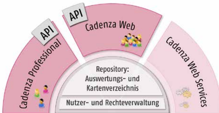
Abbildung 1: Cadenza-Anwendungsrahmen – Architekturschaubild
