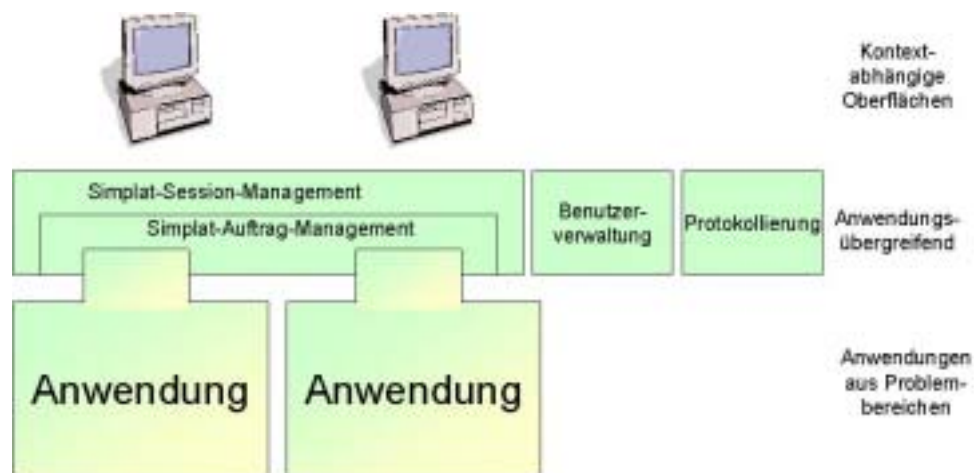
Abbildung 7: Simplat-Architektur, Teil 1
