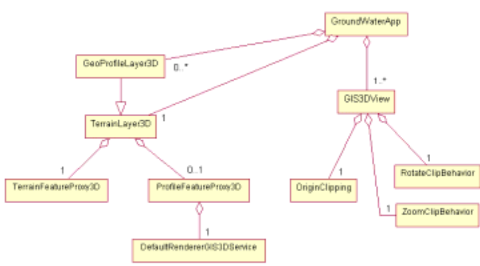
Abbildung 3.6: Klassendiagramm für die 2D-Profilansichten
