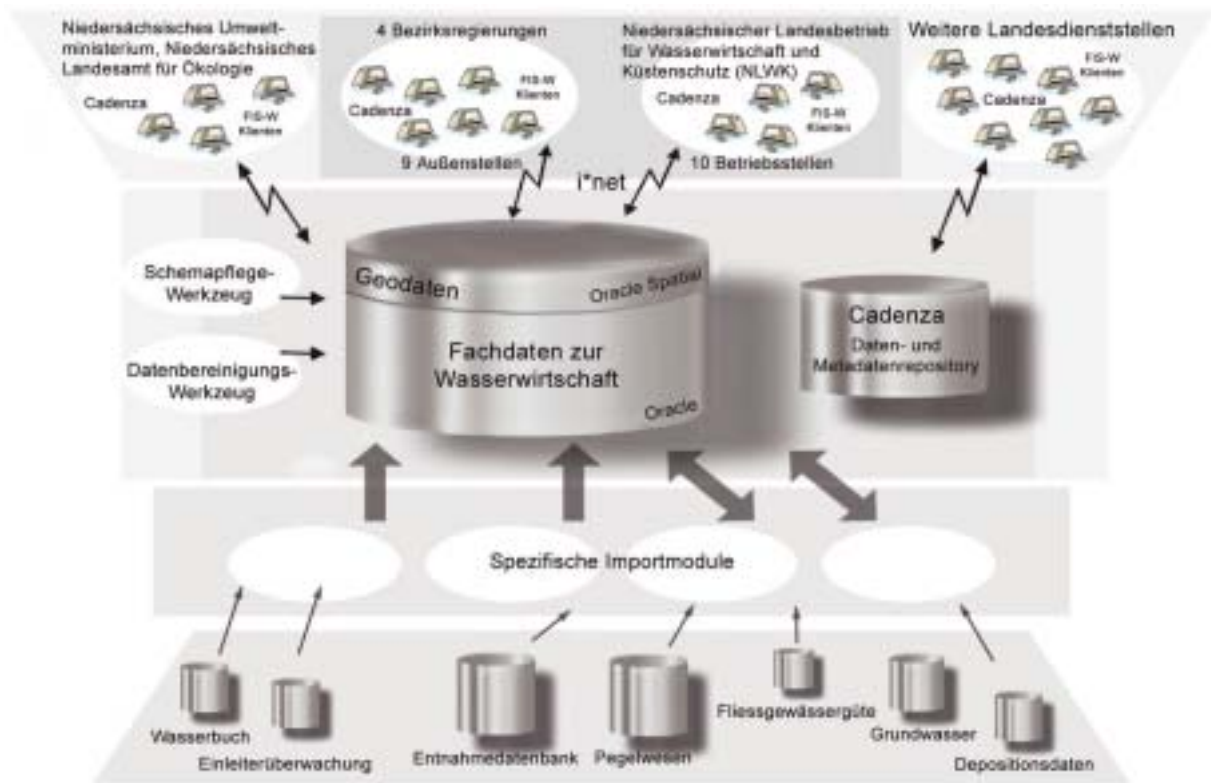
Abbildung 1: Gesamtarchitektur FIS-W
