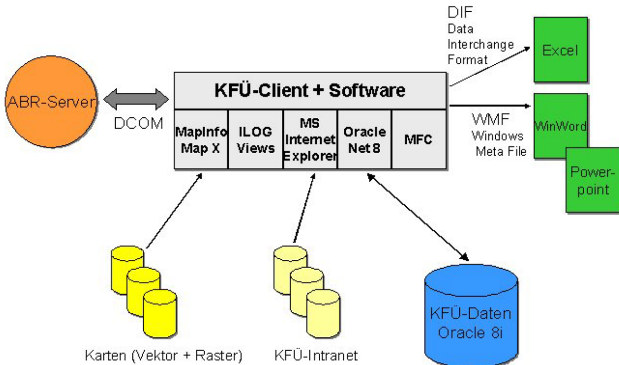
Abbildung 6: Architektur KFÜ-Client
