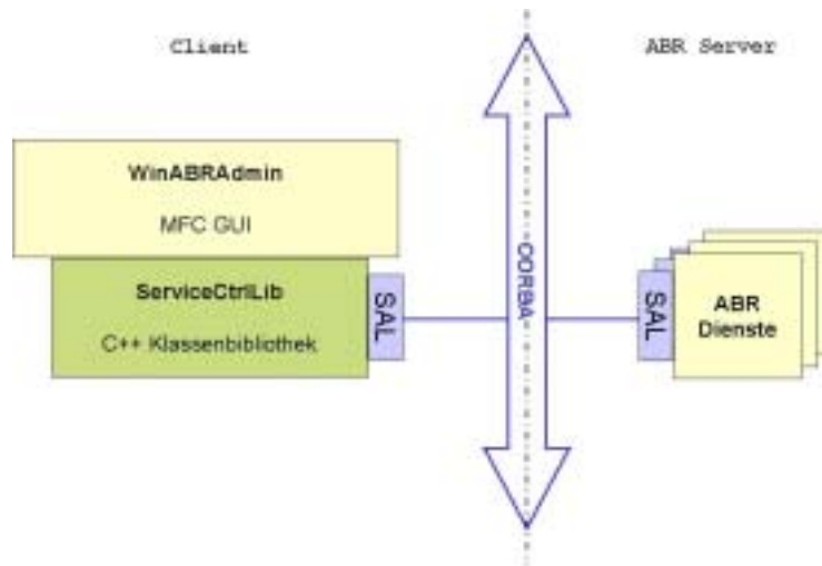
Abbildung 2: Architektur des Dienstes WinABRAdmin
