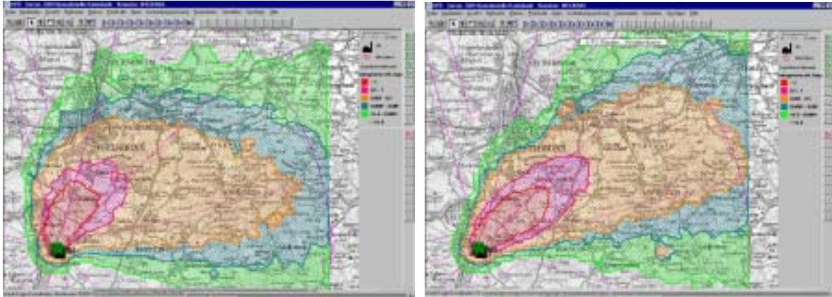
Abbildung 6: Vergleich der eff. Gesamtdosis Erwachsene ermittelt aus Ergebnissen einer prototypischen Ausbreitungsrechnung für den 27.08.02 0:00 (2 Stunden) (Ausgangswerte aus Messung (links) und aus Prognose (rechts))
