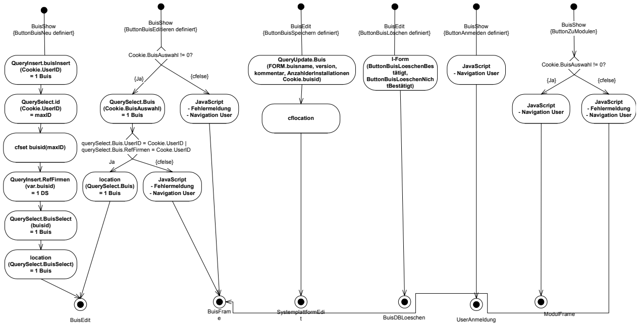
Abbildung 11.5 Ablaufdiagramm „BuisDB“
