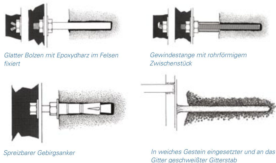
Abbildung 5. Methoden zur Befestigung von Gittern. Wenn Bolzen benutzt werden, sollte das überstehende Ende gespalten, erweitert oder gestaucht werden, damit ein leichtes Abschrauben der Muttern unmöglich ist.
