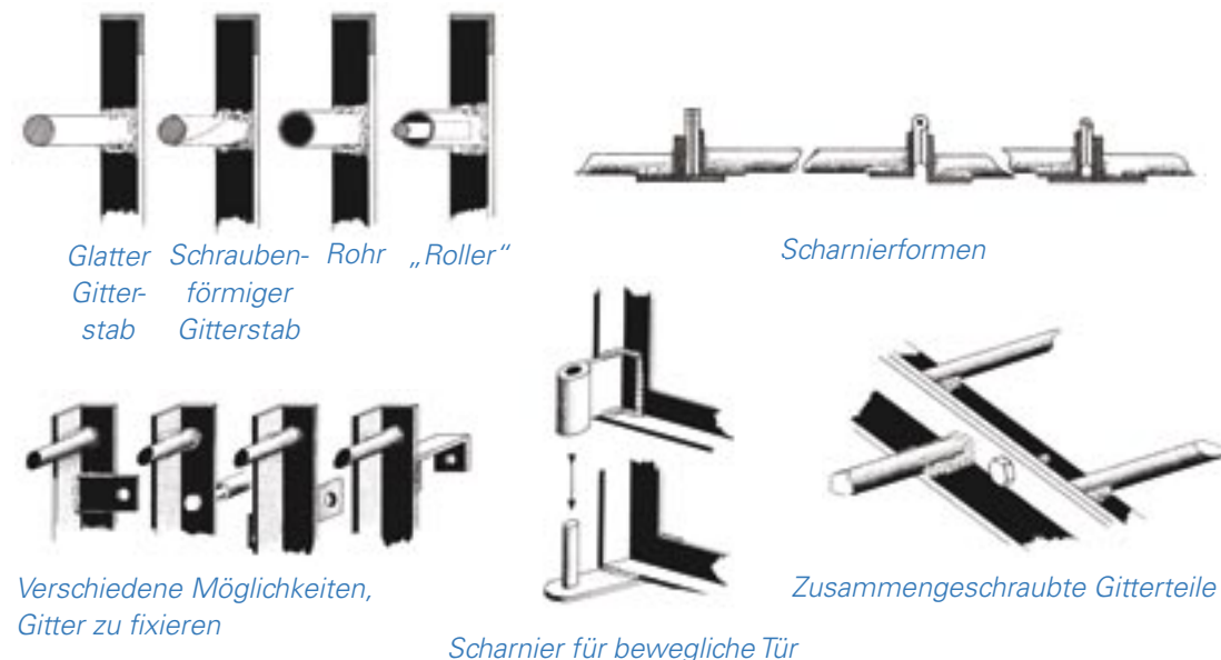
Abbildung 4. Einzelheiten der Gitter
