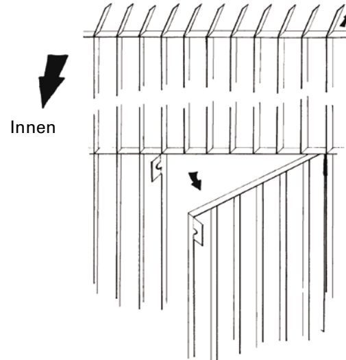
Ausrichtung der Tür und der Zaunspitzen
