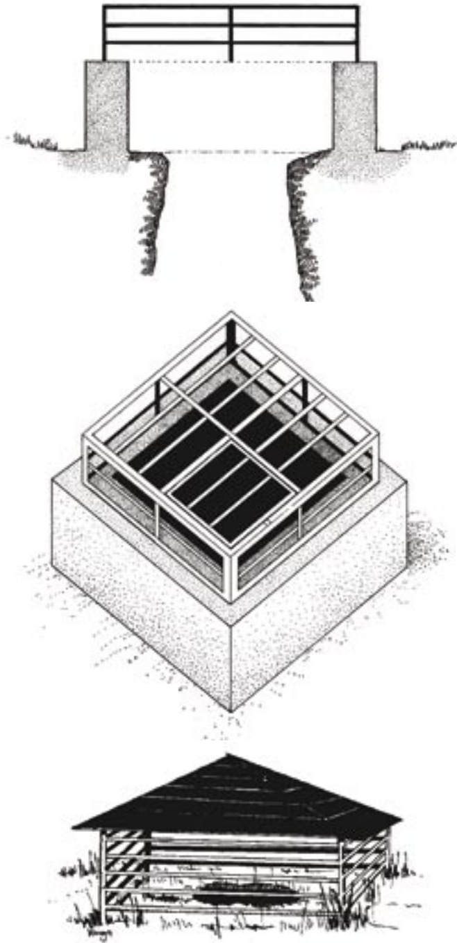
Abbildung 7. Gitter für vertikale Schächte. Horizontale Gitter sollten nicht ebenerdig angebracht werden, weil diese nicht sicher sind und zuwachsen können. Es könnte notwendig sein, das obere Ende einer Höhle oder eines Schachts zu stabilisieren. Fledermäuse scheinen keine Schwierigkeiten zu haben, einen vertikalen Schacht hoch- und durch ein vertikales Gitter hindurch zu fliegen.
