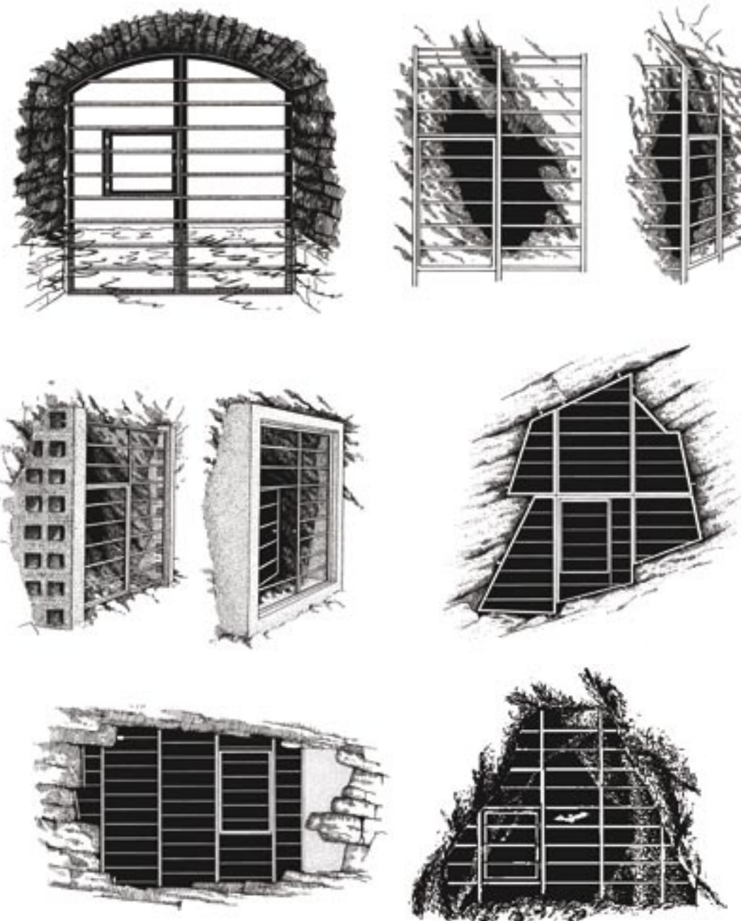
Abbildung 3. Beispiele für Vergitterungen von horizontalen Eingängen. Gitter können so konstruiert sein, dass sie entweder größer sind als der Eingang und davor angebracht werden oder dass sie im Eingangsbereich mit Schrauben bzw. Nägeln befestigt werden. Sie können auch genau in den Zugang eingepasst werden und diesen stabilisieren. Breite Gitter können außerhalb der Stätte in Einzelteilen konstruiert und an der Stätte zusammengeschaubt oder -geschweißt werden. Eine verschließbare Eingangstür sollte immer eingepasst werden.
