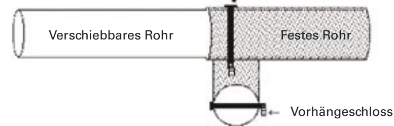
Abbildung 2. Gittergestaltung, wie sie in Frankreich zum Einsatz kommt. Die Rohre sind mit Kies, Stahl und Zement gefüllt, was Sägen einen starken Widerstand entgegen setzt.
