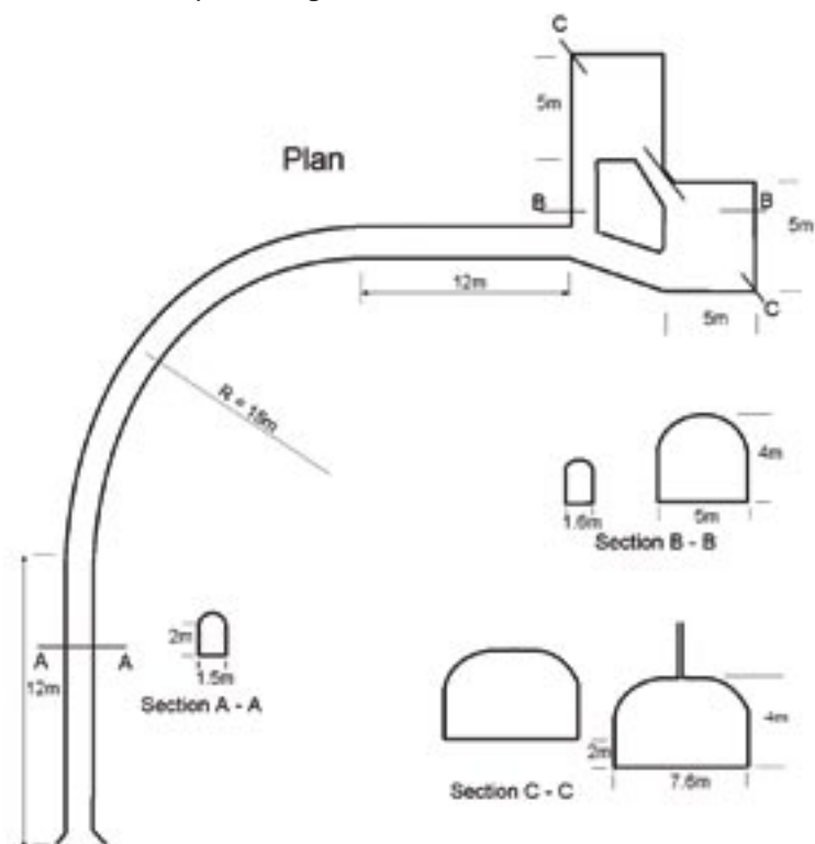
Abbildung 11: Gestaltung der künstlichen Stollen in Portugal.
