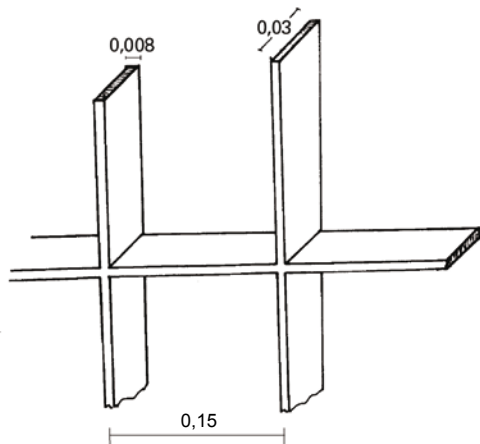
Abstände zwischen den einzelnen Zaunstangen.
