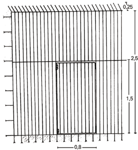
Sicherheitszaun: übliche Ausführung.
