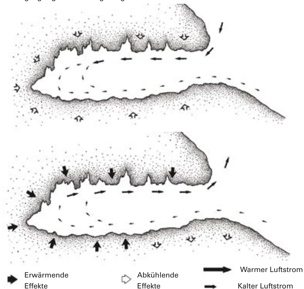
Abbildung 1. Luftströmung in einer unterirdischen Stätte. Die Temperatur tief unter Tage entspricht fast der jährlichen Durchschnittstemperatur der Umgebung. Im Sommer, wenn die Außentemperatur höher ist als die unterirdische, fließt warme Luft in die Höhle, kühlt dort ab, wird dadurch schwerer und fließt bergab (oben). Im Winter ist die Luftströmung umgekehrt, weil kalte Luft angewärmt wird und aufsteigt (unten). Aushöhlungen an der Decke sind stets die wärmsten Plätze im Quartier.
