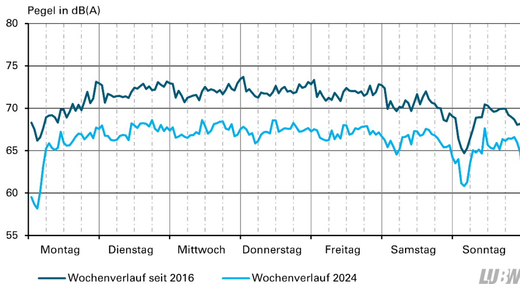
Abbildung 3: Durchschnittlicher Wochenverlauf der Vorbeifahrtpegel im Vergleich mit dem langjährigen Mittel
