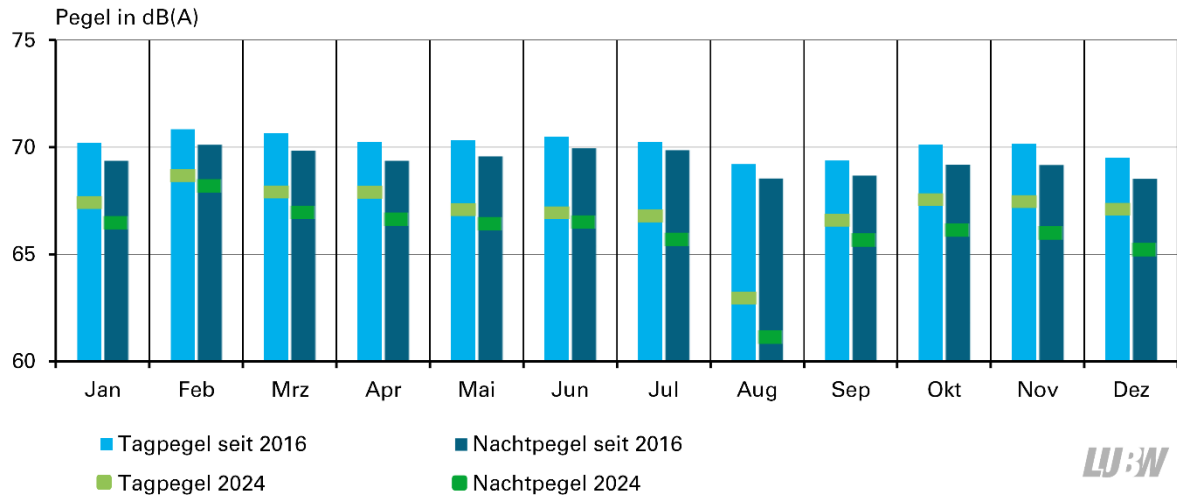
Abbildung 2: Monatsmittelungspegel des Vorbeifahrtgeräusches im Vergleich mit dem langjährigen Mittel
