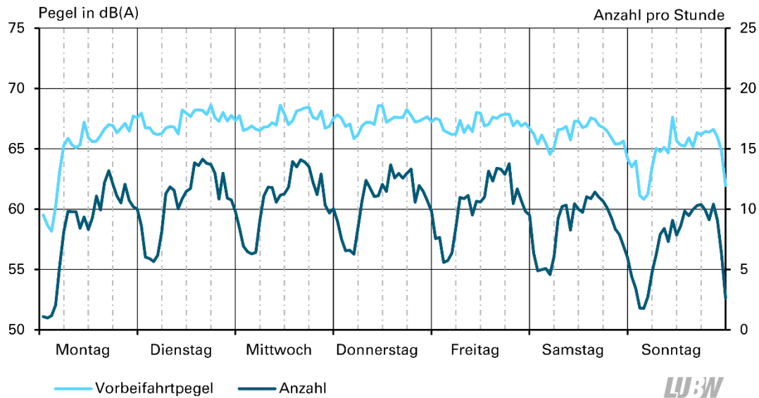
Abbildung 18: Durchschnittlicher Wochenverlauf der Stundenmittelungspegel und der stündlichen Anzahl der Vorbeifahrten
