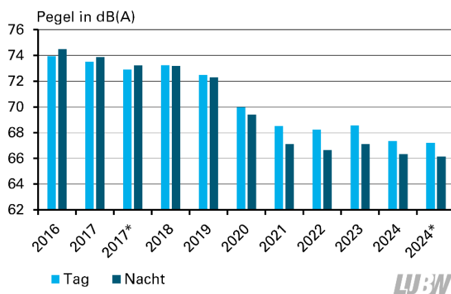
Abbildung 14: Jahresmittelungspegel des Vorbeifahrtgeräusches seit 2016
