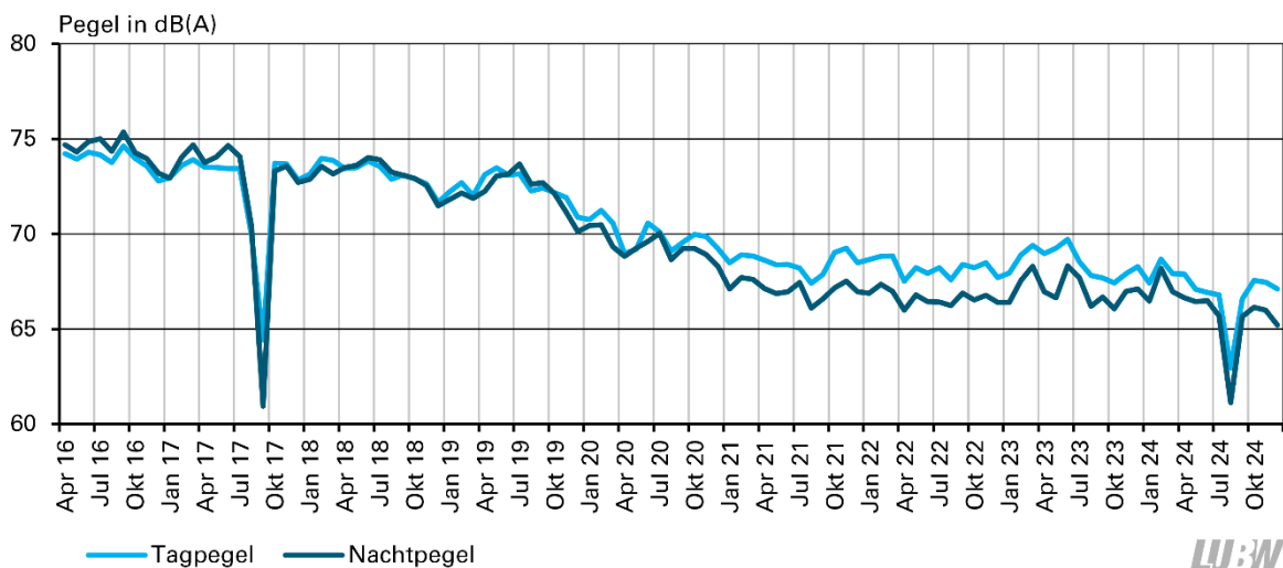
Abbildung 17: Monatsmittelungspegel des Vorbeifahrtgeräusches seit 2016
