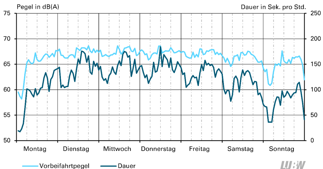
Abbildung 19: Durchschnittlicher Wochenverlauf der Stundenmittelungspegel und der stündlichen Dauer der Vorbeifahrten
