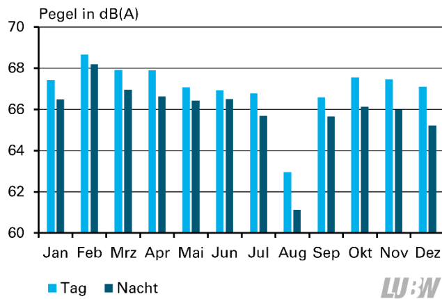
Abbildung 16: Monatsmittelungspegel des Vorbeifahrtgeräusches
