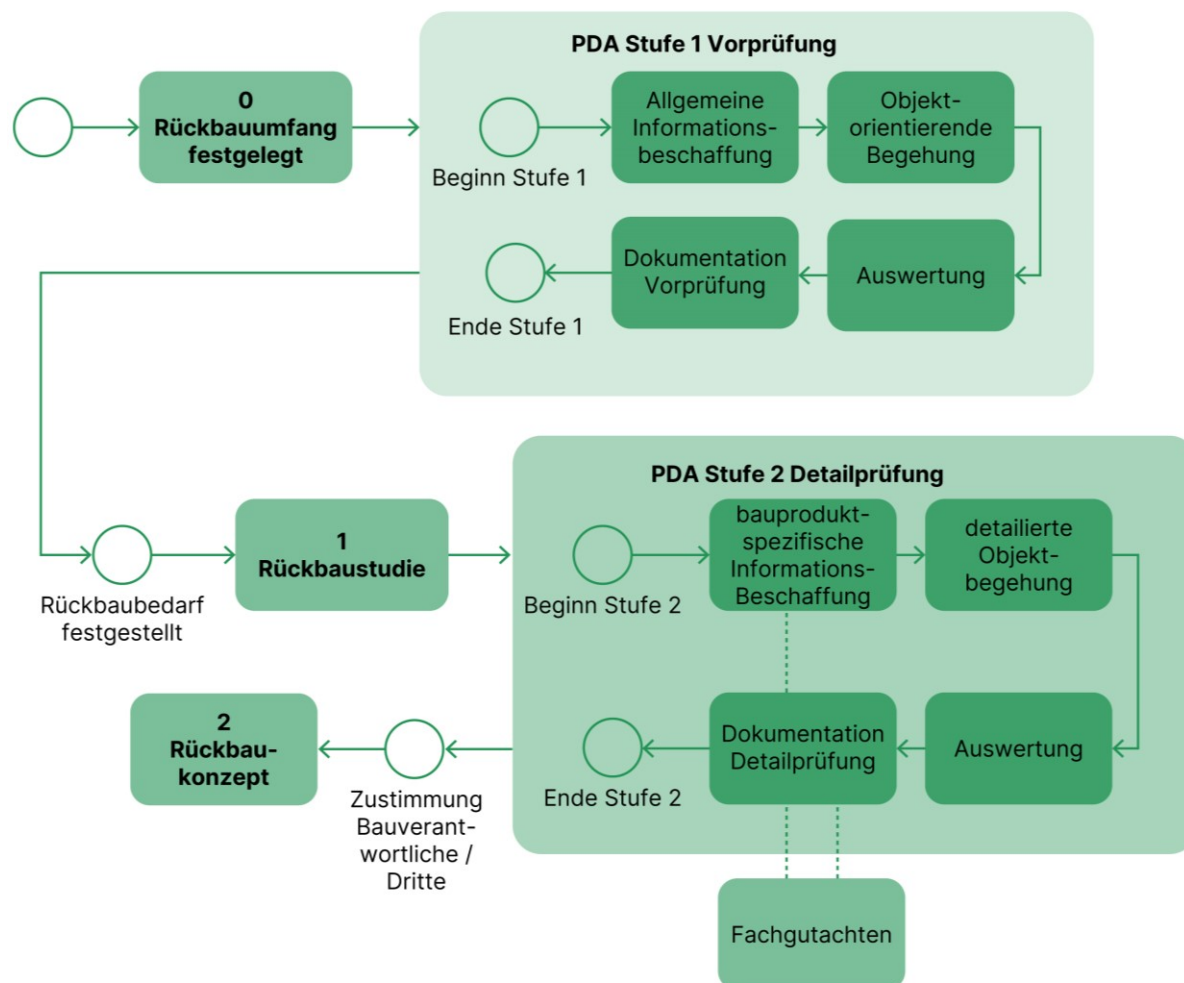
Abbildung 5.4: Prozessablaufdiagramm der Bestandsaufnahme nach DIN SPEC 91484
