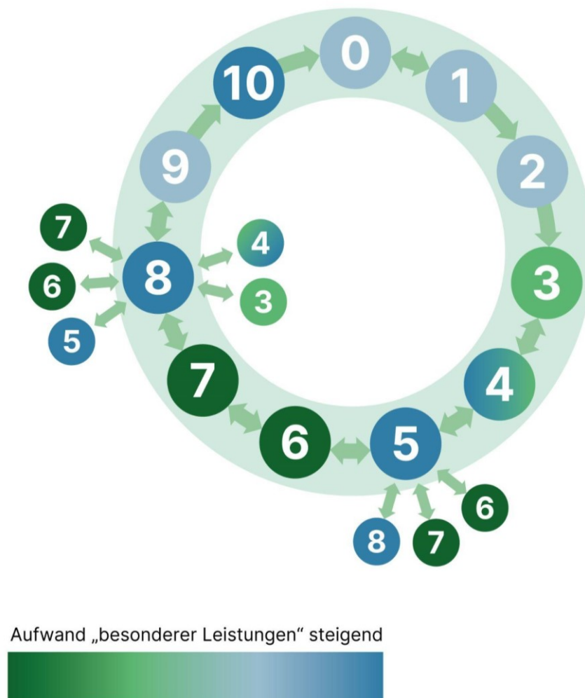
Abbildung 3.1: Zirkuläres Leistungsphasenmodell
