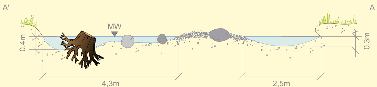
beispielhafter Schnitt mit abgelagerter Kiesbank hinter Totholz
