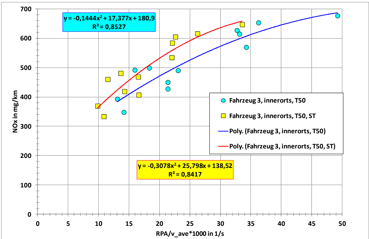
Abbildung 6-42: \text{NO}_x -Emissionen über dem Quotienten aus RPA und mittlerer Geschwindigkeit für Fahrzeug 3
