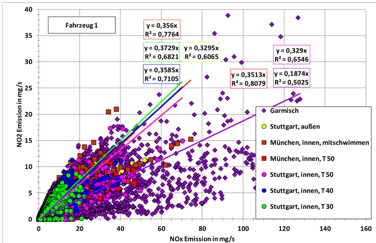
Abbildung 6-59: NO 2 /NO x -Verhältnisse Fahrzeug 1
