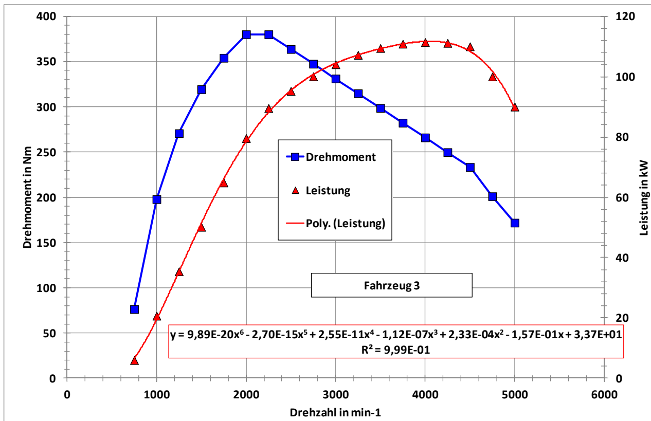
Abbildung 4-11: Motorleistungskurve Mazda 6
