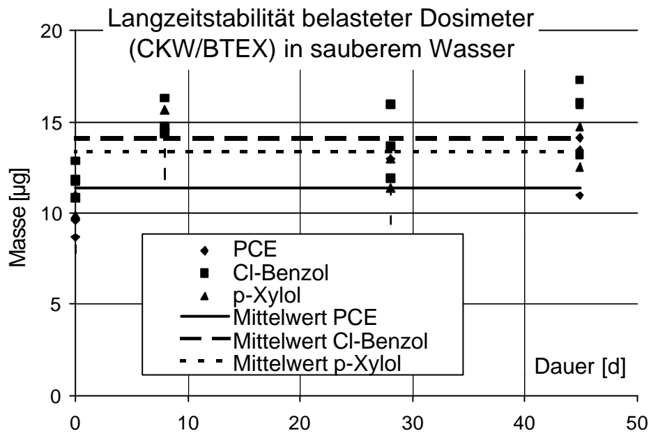
Abb. 4.35: Test der Langzeitstabilität beladener (PCE, Cl-Benzol, pXylol) Keramikdosimeter mit trockenem Adsorbermaterial (5 cm Länge, 5 nm Porengröße) über ca. 45 Tage in sauberem Wasser.
