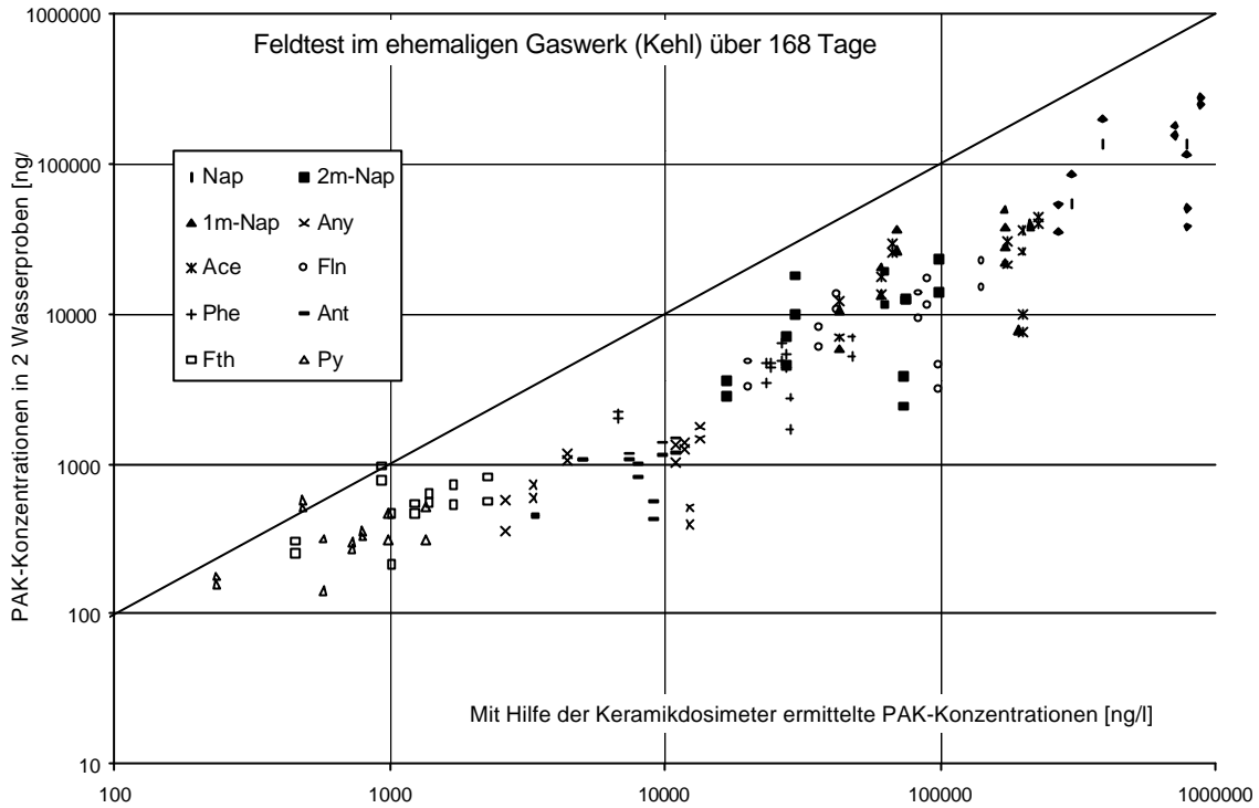
Abb. 4.37: Feldtests der Keramikdosimeter mit wassergesättigtem Adsorbiermaterial (5 cm Länge, 5 nm Porengröße) über 168 Tage in einem Multilevelbrunnen (7 Level) im ehemaligen Gaswerk in Kehl.
