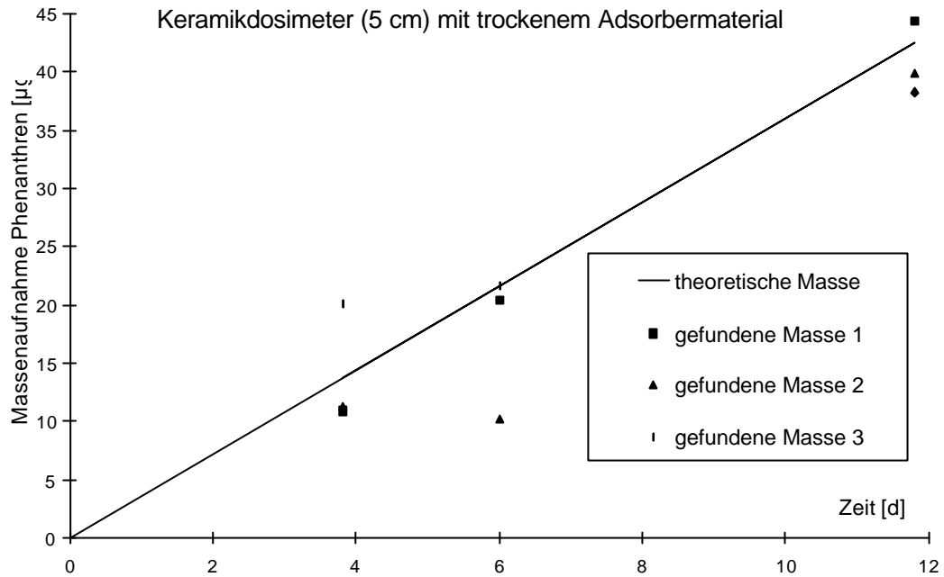
Abb. 4.29: Lineare Aufnahme von Phenanthren im Keramikdosimeter mit trockenem Adsorbentmaterial (5 cm Länge, 5 nm Porengröße) über fast 12 Tage. Die durchgezogene Linie stellt die berechnete kumulative Aufnahme nach Gl. 2-4 dar (Piepenbrink, 1998) ( \epsilon = 30,5\% ; m = 2 ; D_w = 6,71 \cdot 10^{-6} \text{ cm}^2 \text{ s}^{-1} ; D_g = 0,0597 \text{ cm}^2 \text{ s}^{-1} ; C_w = 1,2 \text{ µg cm}^{-3} ; C_g = 0 \text{ µg cm}^{-3} ; Z_w = 0,15 \text{ cm} ; Z_g = 0,01 \text{ cm} ; H = 0,001 ; A = 8,35 \text{ cm}^2 ).
