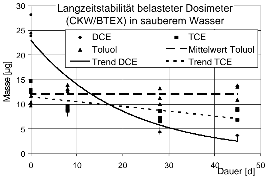
Abb. 4.36: Test der Langzeitstabilität beladener (DCE, TCE, Toluol) Keramikdosimeter mit trockenem Adsorbermaterial (5 cm Länge, 5 nm Porengröße) über ca. 45 Tage in sauberem Wasser.
