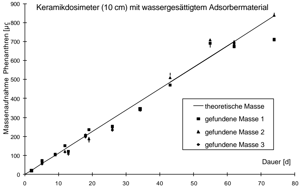
Abb. 4.31: Lineare Aufnahme von Phenanthren im Keramikdosimeter mit wassergesättigtem Adsorbiermaterial (10 cm Länge, 100 nm Porengröße) über mehr als 70 Tage. Die durchgezogene Linie stellt die berechnete kumulative Aufnahme nach Gl. 2-3 dar ( \epsilon = 31,9\% ; m = 1,7 ; D_e = 1,12 \cdot 10^{-6} \text{ cm}^2 \text{ s}^{-1} ; DC = 1,2 \mu\text{g cm}^{-3} ; Dx = 0,15 \text{ cm} ; A = 17 \text{ cm}^2 ).
