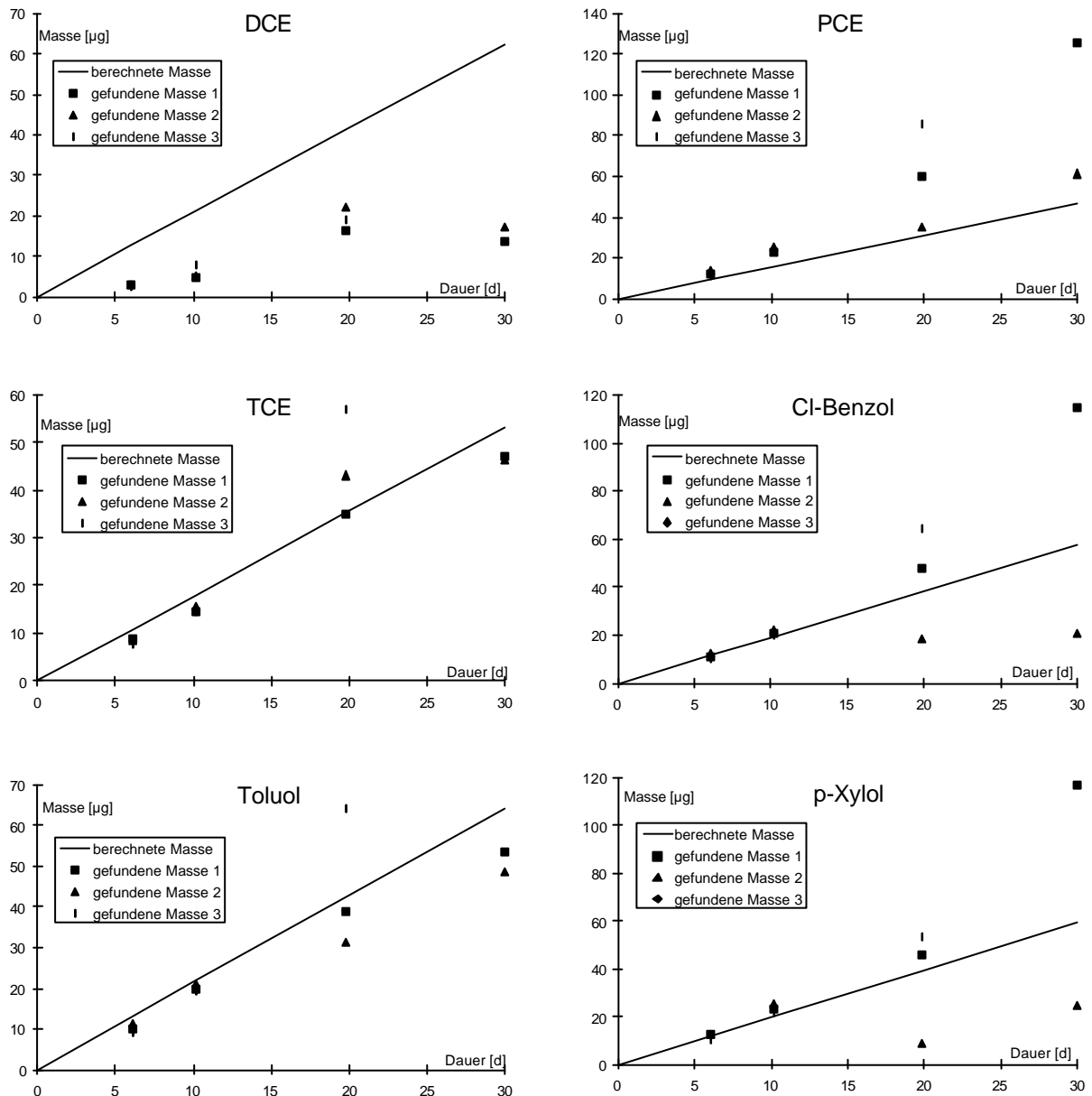
Abb. 4.33: Aufnahme von CKW und BTEX in Keramikdosimeter mit trockenem Adsorbentmaterial (5 cm Länge, 5 nm Porengröße) über 30 Tage. Die durchgezogene Linie stellt die berechnete kumulative Aufnahme nach Gl. 2-4 dar e = 30,5\% ; m = 2 ; D_w , D_g und H , s. Tab. 3.5; Z_w = 0,03 cm; Z_g = 0,1 cm; DC = 0,1 \mu\text{g cm}^{-3} (die während der Eichung gemessenen Wasserkonzentrationen wurden auf eine einheitliche Konzentration normiert und die Messwerte entsprechend korrigiert); A = 8,35 \text{ cm}^2 . Oben links DCE, rechts PCE, Mitte links TCE, rechts Cl-Benzol, unten links Toluol, rechts p-Xylol.
