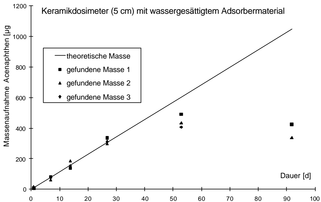
Abb. 4.32: Aufnahme von Acenaphthen in Keramikdosimeter mit wassergesättigtem Adsorbiermaterial (5 cm Länge, 5 nm Porengröße) über mehr als 90 Tage. Die durchgezogene Linie stellt die berechnete kumulative Aufnahme nach Gl. 2-3 dar ( \epsilon = 30,5\% ; m = 2 ; D_e = 6,79 \cdot 10^{-7} \text{ cm}^2 \text{ s}^{-1} ; Dx = 0,15 \text{ cm} ; DC = 3,5 \mu\text{g cm}^{-3} ; A = 8,35 \text{ cm}^2 ).
