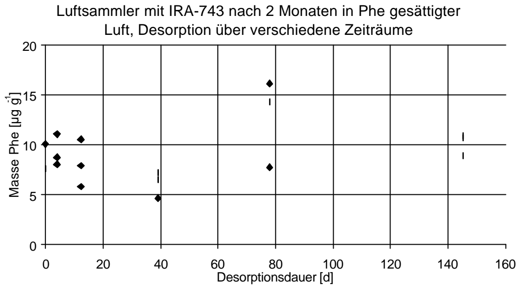
Abb. 4.28: Desorptionstest von mit Phenanthren belasteten Adsorbermaterial.
