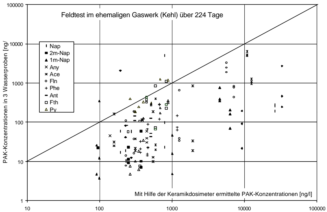
Abb. 4.38: Feldtests der Keramikdosimeter mit wassergesättigtem Adsorbiermaterial (5 cm Länge, 5 nm Porengröße) über 224 Tage in einem Multilevelbrunnen (7 Level) im ehemaligen Gaswerk in Kehl.
