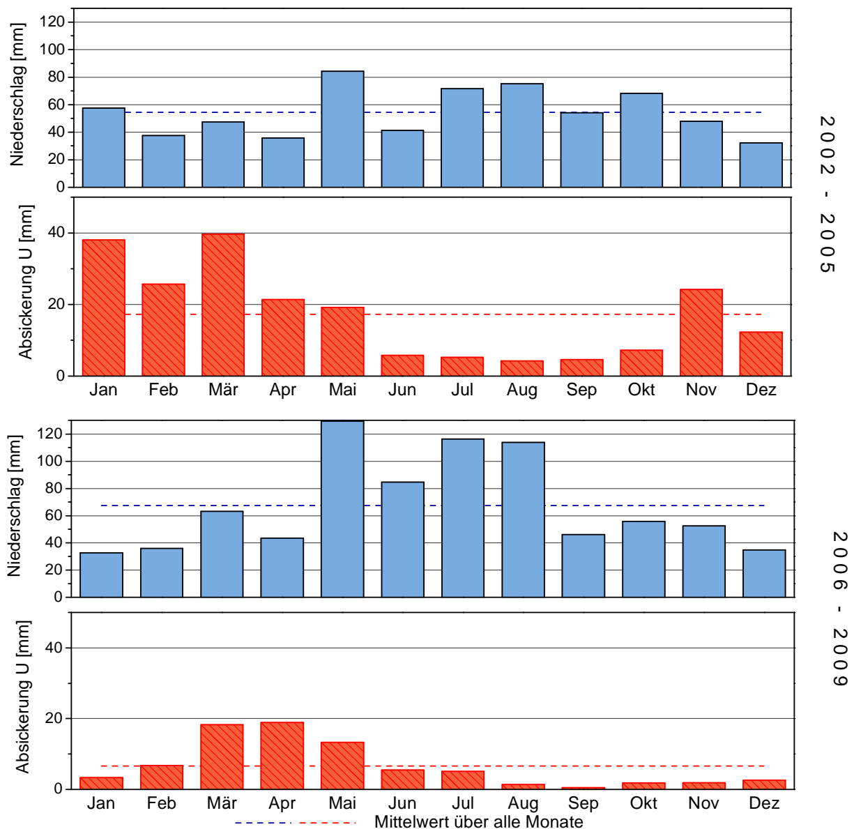
Abbildung 3-15: Mittlere Monatssummen [mm] von Niederschlag und Absickerung aus dem U-Feld in den Jahren 2002 - 2005 (oben) und 2006 - 2009 (unten)
