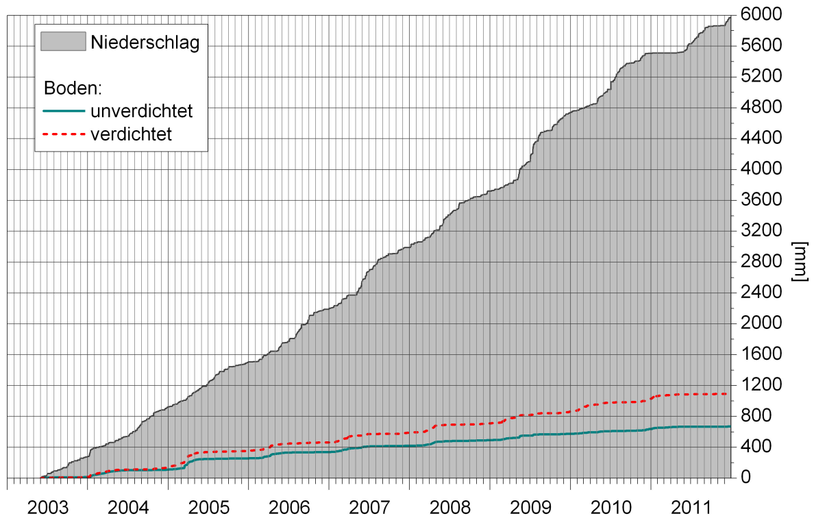
Abbildung 3-13: Niederschlag in Leonberg und Absickerung aus den Lysimeterfeldern U (Boden unverdichtet) und K (Boden verdichtet) von Juni 2003 bis Dezember 2011
