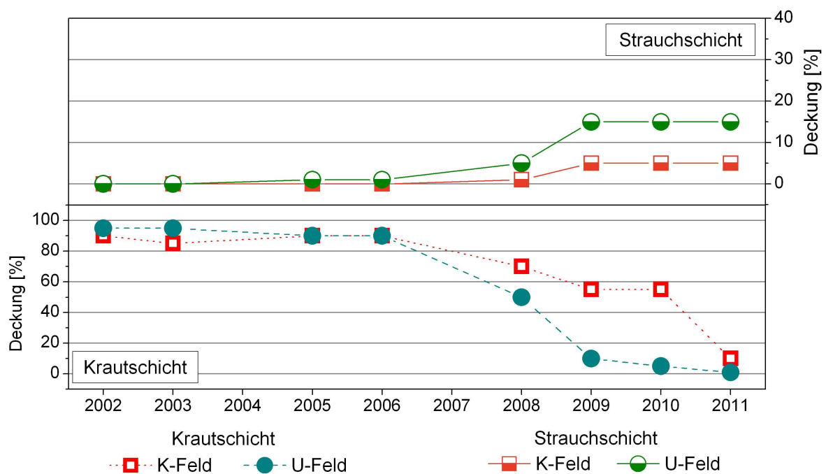
Abbildung 3-12: Deckungsgrade [%] der Kraut- und Strauchschicht in je 40 m 2 großen Vegetations-Aufnahmeparzellen in den Testfeldern U und K
