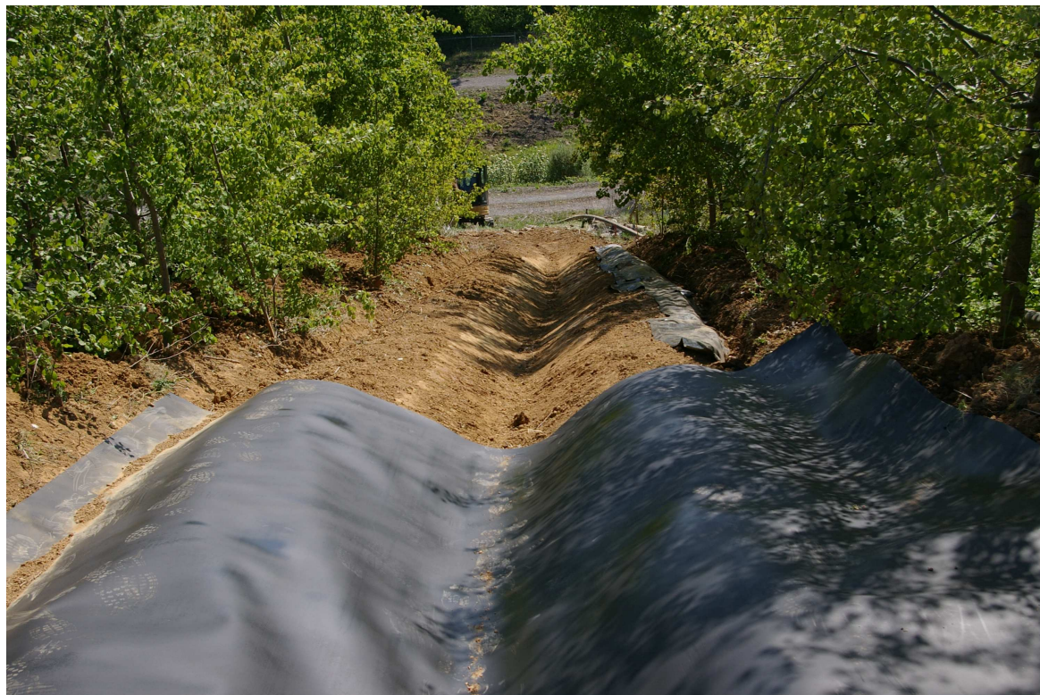
Bild 2: Reparaturarbeiten im Mai 2008: neu profiliertes und mit HDPE-Folie belegter Trennstreifen
