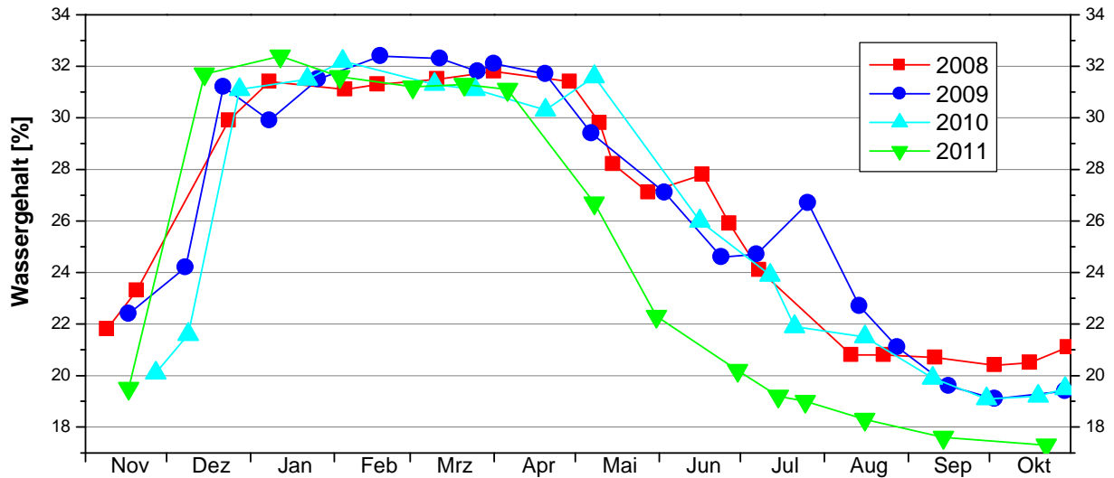
Abbildung 3-6: Verlauf der Wassergehalte des Unterbodens (85 cm Tiefe) des U-Feldes im Jahr 2011 im Vergleich zu den Vorjahren 2008 – 2010.
