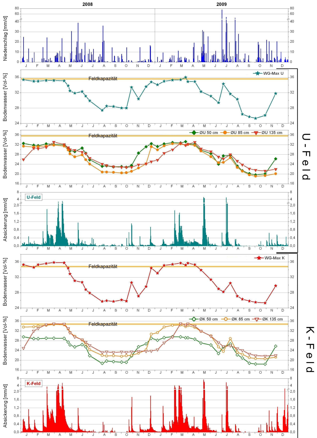
Abbildung 3-16: Niederschlag, mittlere ( \varnothing in 50, 85 und 135 cm Tiefe) und maximale (WG-Max) Bodenwassergehalte und Feldkapazität des Bodens sowie Absickerung, U- und K-Feld, Tageswerte vom 1.1.2008 bis 31.12.2009
