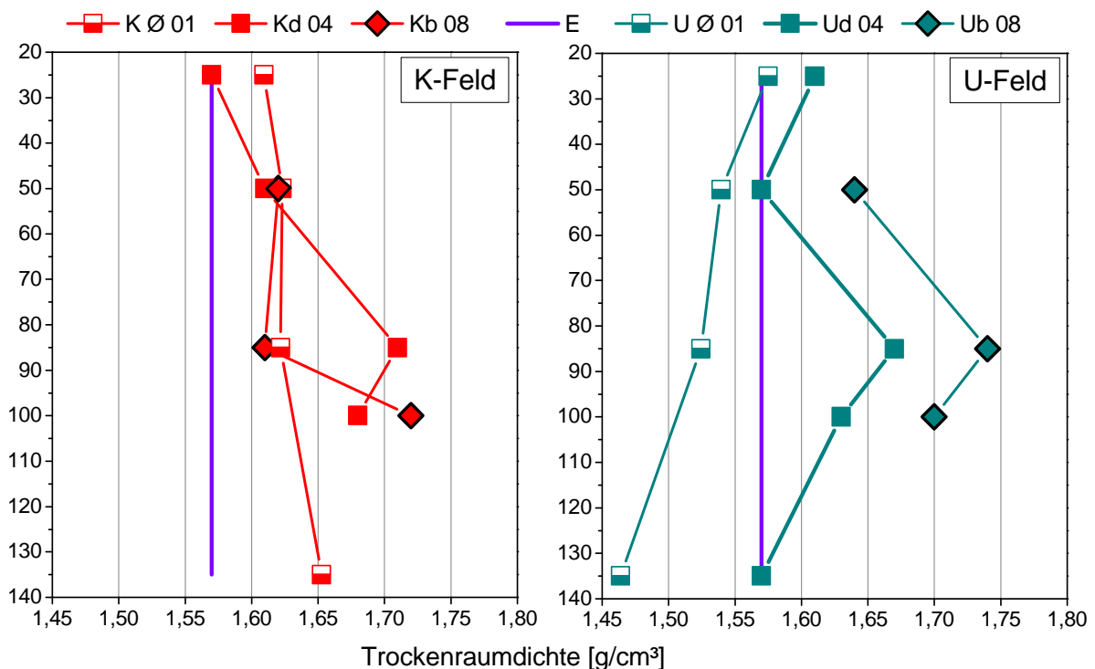
Abbildung 3-4: Trockenraumdichten in den Jahren 2001 (Ø 01 = Mittel von 4 Probestellen), 2004 und 2008; die Kleinbuchstaben geben die Lage im Testfeld an: b = Unterhang, d = Oberhang, E = mittlere Dichte des Bodenmaterials im Einbauzustand
