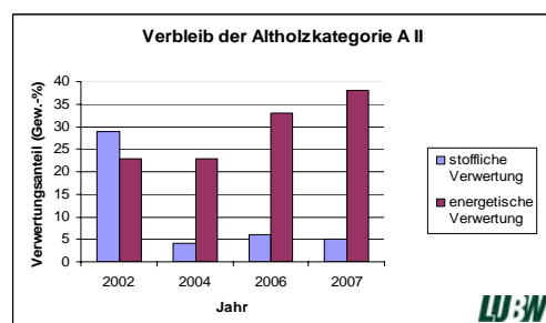
Abb. 14: Anteil der Altholzkategorie A II an der stofflichen und energetischen Verwertung (Gew.-%)
