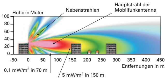
Abb. 12.3-7: Beispiel für das Abstrahlverhalten einer Mobilfunkantenne (Sektorantenne in 30 m Höhe). Die angegebenen Werte beziehen sich auf die Leistungsflussdichte (in Milliwatt pro m 2 ). Quelle: LfU Bayern 2009
