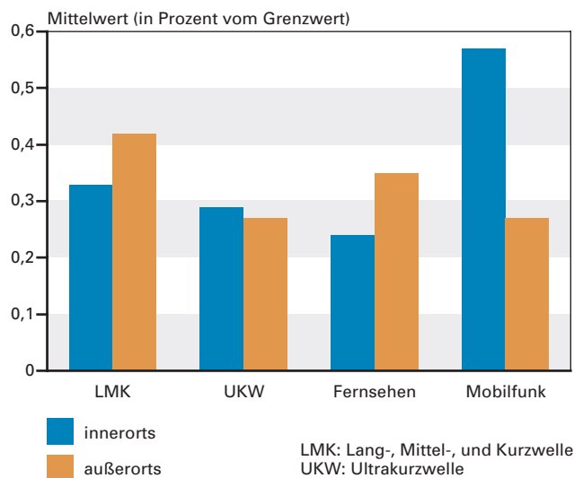
Abb. 12.3-1: Beiträge von Rundfunk, Fernsehen und Mobilfunk innerorts und außerorts im Vergleich – dargestellt sind die erreichten Prozentanteile des Grenzwertes [LFU 2003].
