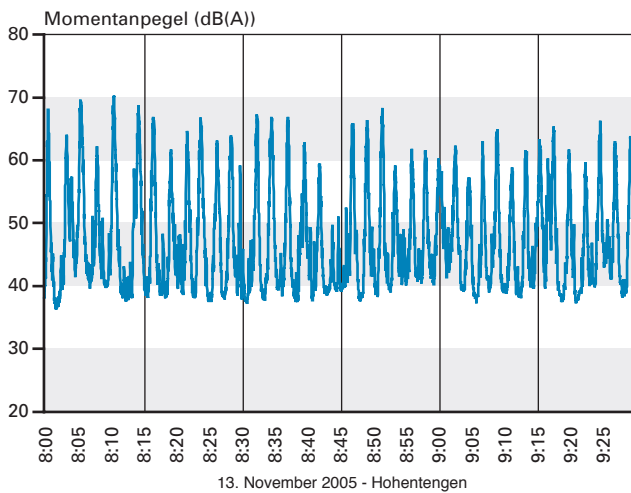
Abb. 5.3-11: Fluglärm – typischer Pegel-Zeitverlauf am Tag (Hohentengen, 13.11.2005 ab 8.00 Uhr bis 9.30 Uhr). Quellen: Landkreis Waldshut, LUBW. Stand: 2005
