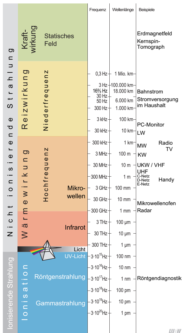
Abb. 12.1-1: Der physikalische Begriff der elektromagnetischen Welle (bzw. Felder oder Strahlen) umfasst einen weiten Frequenzbereich – hier mit Beispielen technischer Nutzung.
