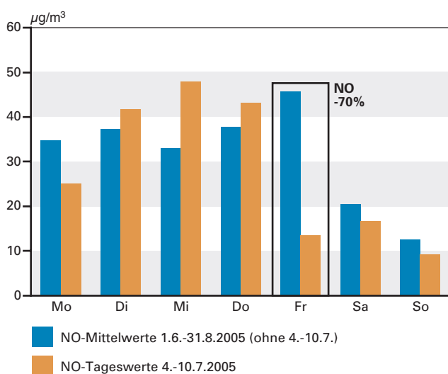
Abb. 4.2-7: Auswirkung einer 12-stündigen Straßensperrung auf die Luftschadstoffkonzentrationen an der Station ‚Karlsruhe-Straße‘. Linke Säulen: Mittlere Konzentration für die Wochentage im Sommerquartal (1.6.-31.8.2005); rechte Säulen: Tageswerte in der Woche 4.-10.7.2005. Die Straßensperrung war am Freitag, dem 8.7.2005 [LUBW 2008b].
