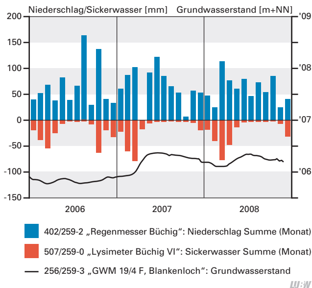
Abb. 6.1-11: Niederschlag, Sickerung und Grundwasserstand an der Lysimeteranlage Büchig. Stand: 2009
