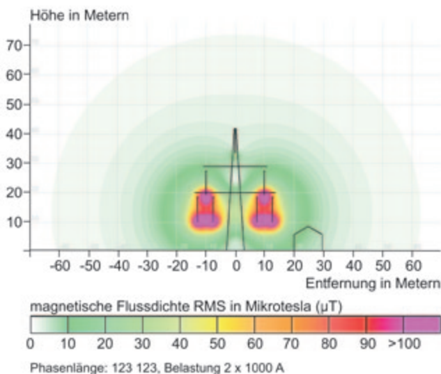
Abb. 12.3-4: Verlauf der magnetischen Flussdichte in der Umgebung einer 380-kV-Freileitung. Quelle: WinField, Forschungsgesellschaft für Energie und Umwelttechnologie – FGEU 2009
