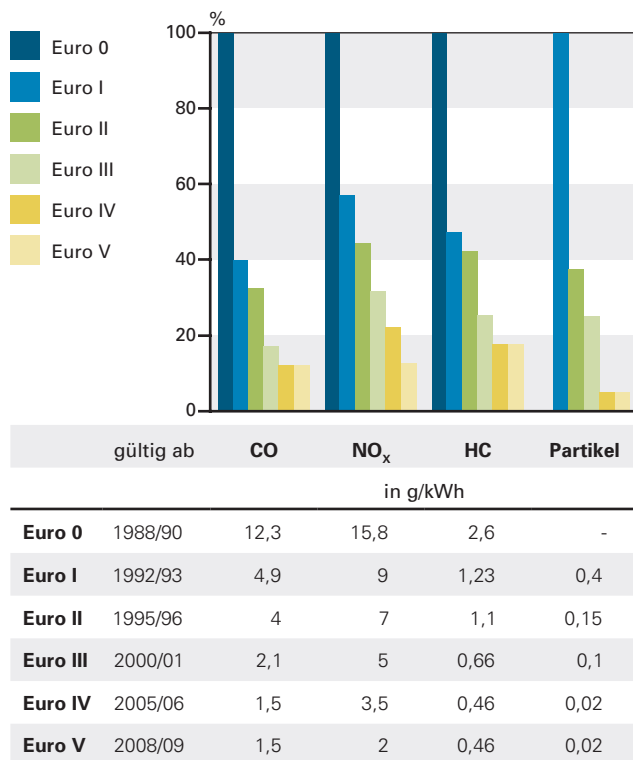
Abb. 4.2-10: Entwicklung der europäischen Abgasgrenzwerte für schwere Nutzfahrzeuge über 3,5 t Gesamtgewicht. Abgasgrenzwerte in g/kWh. Quelle: EU, Umweltbundesamt
