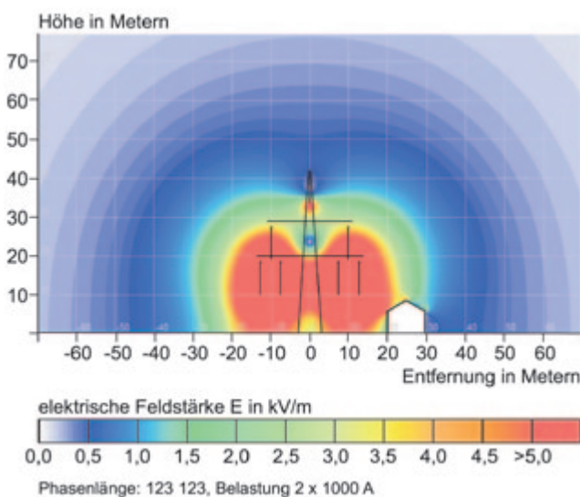
Abb. 12.3-3: Verlauf der elektrischen Feldstärke in der Umgebung einer 380-kV-Freileitung. Quelle: WinField, Forschungsgesellschaft für Energie und Umwelttechnologie – FGEU 2009
