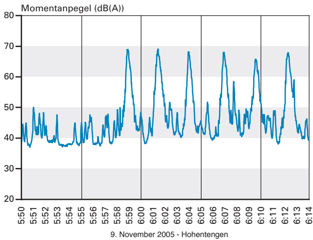
Abb. 5.3-10: Fluglärm – typischer frühmorgendlicher Pegel-Zeitverlauf (Hohentengen, 9.11.2005 ab 5.50 Uhr bis 6.14 Uhr). Quellen: Landkreis Waldshut, LUBW. Stand: 2005
