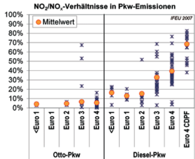
Abb. 4.2-4: Prozentualer NO 2 -Anteil an der NO x -Emission, Einzelmessungen bei Pkw (Innerortszyklus). CDPF = Katalytisch beschichteter Dieselpartikelfilter [IFEU 2007].
