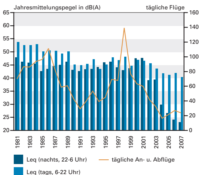
Abb. 5.3-9: Jahresmittelungspegel (Leq = energieäquivalenter Mittelungspegel) und Mittelwert der täglichen Flugzahlen an der Fluglärmmessstation Hohentengen-Herdern. Quelle: Landkreis Waldshut, LUBW. Stand: 2008
