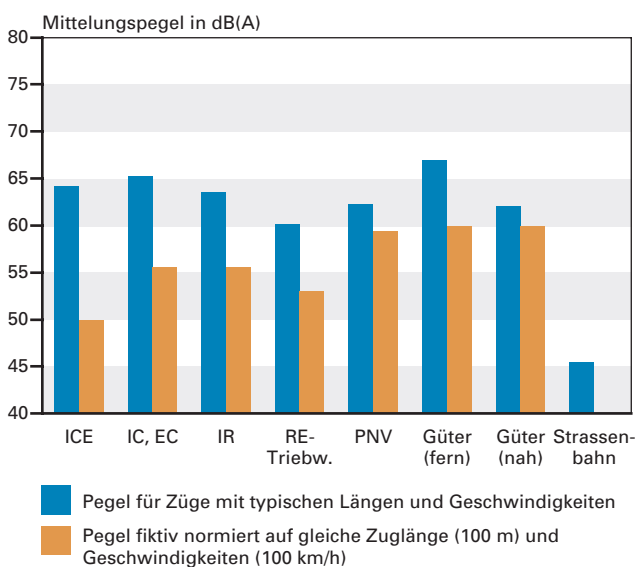
Abb. 5.3-5: Mittelungspegel für verschiedene Zugarten der Deutschen Bahn AG im Vergleich (25 m Abstand, 1 Zug pro Stunde.) Quelle: Deutsche Bahn AG, LUBW. Stand: 2005.
