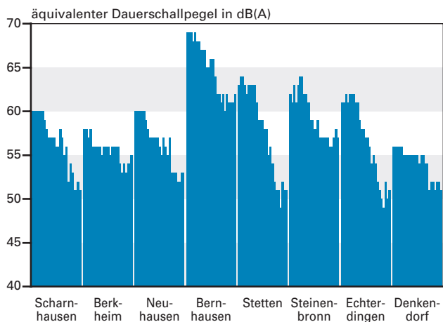
Abb. 5.3-6: Äquivalenter Dauerschallpegel an den Fluglärmmessstationen im Einwirkungsbereich des Flughafens Stuttgart 1982-2006 [FLUGLÄRMSCHUTZBEAUFTRAGTER 2007].
