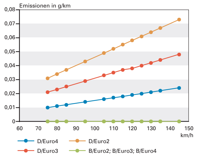
Abb. 4.2-6: Partikel-Emissionsfaktoren differenziert nach Fahrzeugkategorien und Emissionskonzepten (D=Diesel-Pkw, B=Benzin-Pkw) [HBEFA 2004].
