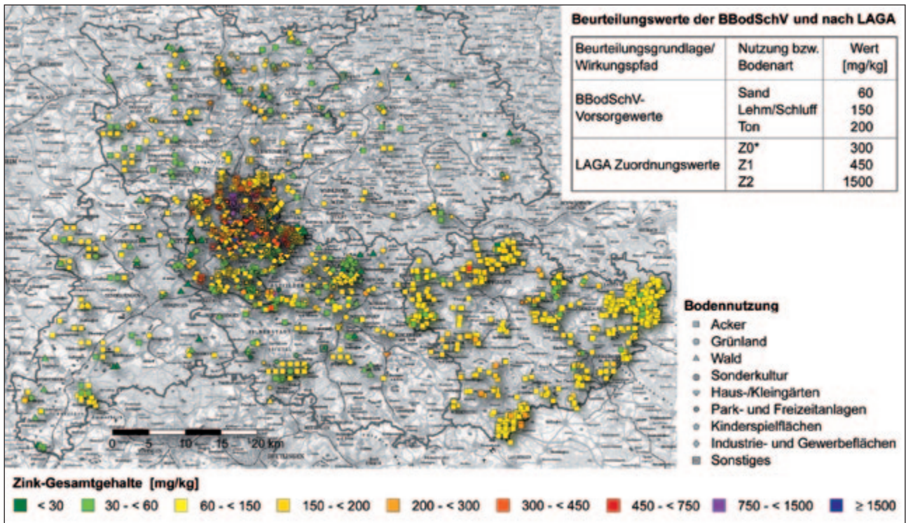
Abb. 7.3-1: Zink-Gehalte im Oberboden in der Region Stuttgart. Quelle: LUBW/Verband Region Stuttgart 2009
