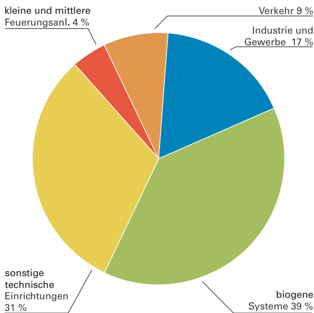
Abb. 4.1-13: Verteilung der NMVOC-Emissionen auf die Quellengruppen in Baden-Württemberg 2006. Stand: 2008
