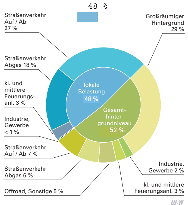
Abb. 4.3-24: Verursacher der Feinstaub PM10-Immissionsbelastung am Messpunkt ‚Stuttgart-Am Neckartor‘ im Jahr 2008. Stand: 2009
