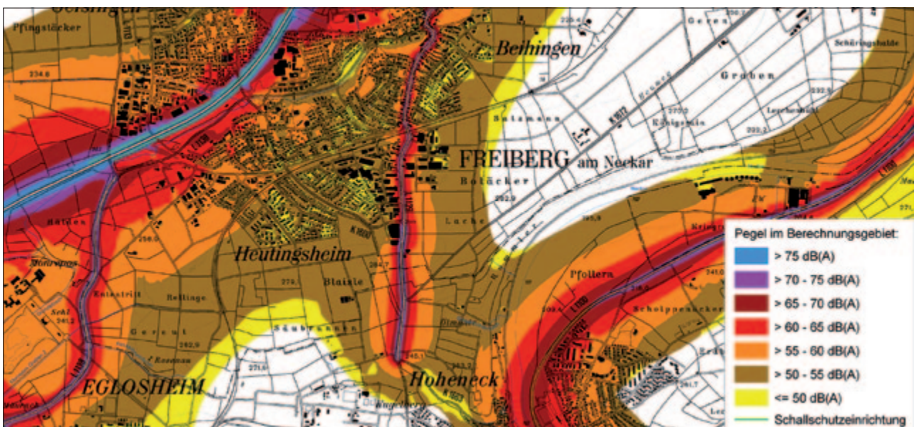
Abb. 5.2-2: Ausschnitt aus einer Lärmkarte für Straßenlärm (L DEN ). Stand: 2007
