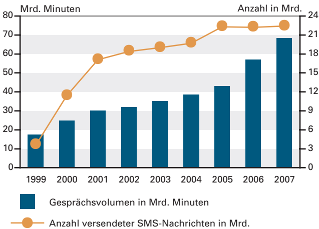
Abb. 12.3-6: Mobilfunknutzung – Entwicklung der Gesprächszeiten (von Mobilfunkgeräten abgehende Gespräche) und SMS-Nachrichten in Deutschland von 1999 bis 2007. Quelle: Bundesnetzagentur 2009
