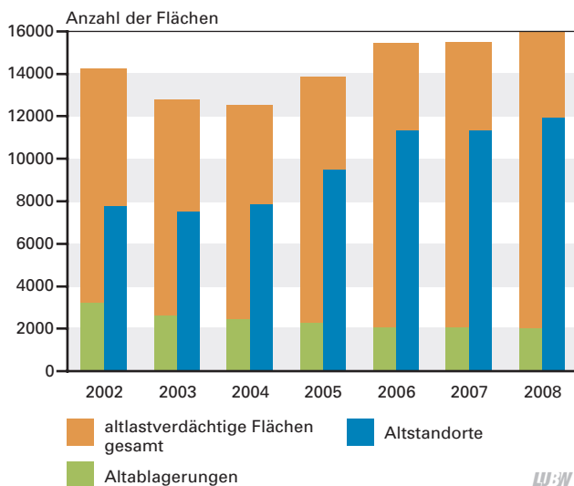
Abb. 13.1-2: Entwicklung der Zahl der altlastverdächtigen Flächen zwischen 2002 und 2008. Stand: 12/2008
