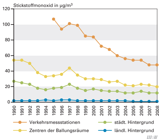
Abb. 4.3-5: Entwicklung der Jahresmittelwerte von NO in Baden-Württemberg von 1990 bis 2008. Stand: 2009
