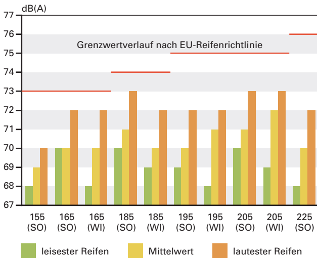
Abb. 5.3-1: Vergleich der Lärmgrenzwerte für Reifen nach der EU-Reifenrichtlinie aus dem Jahr 2001 mit Emissionswerten tatsächlich auf dem Markt befindlicher Reifen [LFU 2004b].
