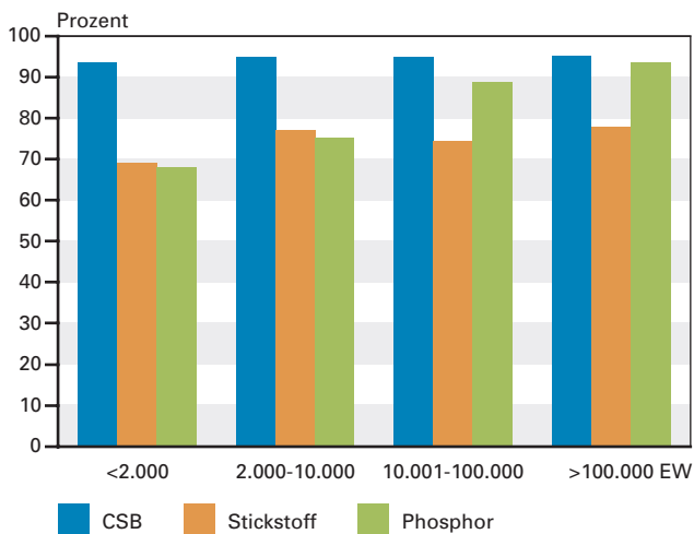
Abb. 6.5-1: Abbau der CSB (Chemischer Sauerstoffbedarf), Stickstoff- und Phosphorfracht unterschiedlich großer Kläranlagen (EW = Einwohnerwert). Stand: 31.12.2008. Quelle: Informationssystem Wasser, Immissionsschutz, Boden, Abfall, Arbeitsschutz (WIBAS)
