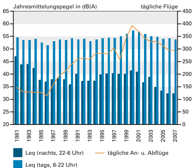
Abb. 5.3-8: Jahresmittelungspegel (Leq = energieäquivalenter Mittelungspegel) und Mittelwert der täglichen Flugzahlen an der Fluglärmmessstation Hohentengen. Quelle: Landkreis Waldshut, LUBW. Stand: 2008
