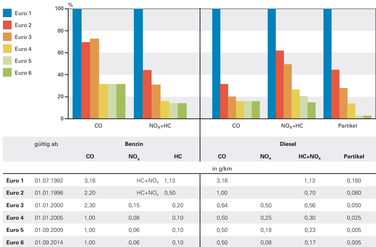
Abb. 4.2-9: Entwicklung der europäischen Abgasgrenzwerte für Otto- und Diesel-Pkw. Abgasgrenzwerte in g/km. Quelle: EU, Umweltbundesamt
