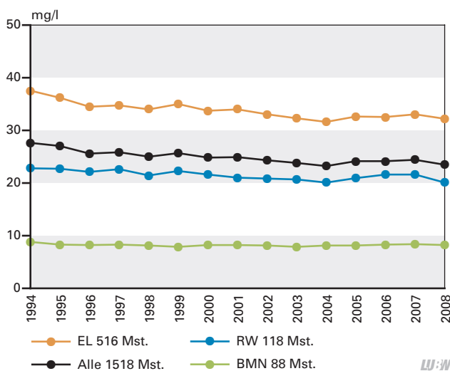
Abb. 6.1-3: Mittelfristige Trends der mittleren Nitratkonzentrationen für jährlich im Herbst beprobte Messstellengruppen – Gesamtsituation innerhalb und außerhalb von Wasserschutzgebieten; EL – Einflussbereich Landwirtschaftliche Nutzung; Alle – alle Landesmessstellen; RW – Rohwasser; BMN – Teilmessnetz Hintergrundkonzentration; Mst. – Messstellen; Daten: Landesmessstellen. Stand: 2009
