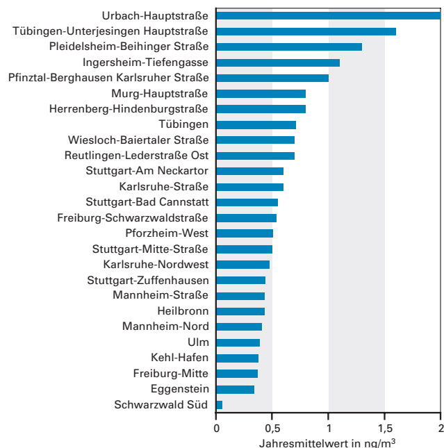
Abb. 4.3-18: Jahresmittelwerte der Konzentration von BaP als Inhaltsstoff des Feinstaubs PM10 für das Jahr 2008 an Messstellen und Spotmesspunkte in Baden-Württemberg. Stand: 2009
