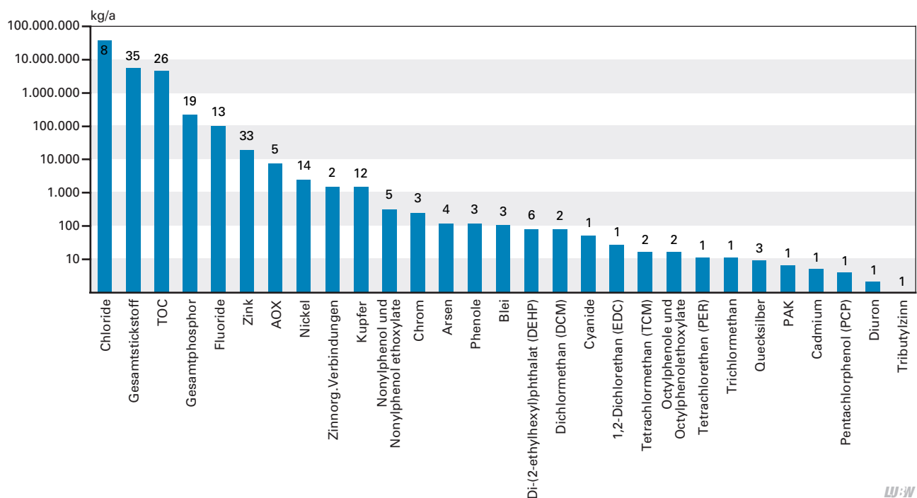
Abb. 6.5-5: Frachten kommunaler Kläranlagen > 100 000 Einwohnerequivalenten und Anzahl der Betriebseinrichtungen im Jahr 2007 in Baden-Württemberg. Stand: 2008
