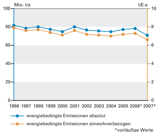
Abb. 1.1-1: Kohlendioxidemissionen. Quelle: Länderarbeitskreis Energiebilanzen 2009, Statistisches Landesamt Baden-Württemberg 2009
