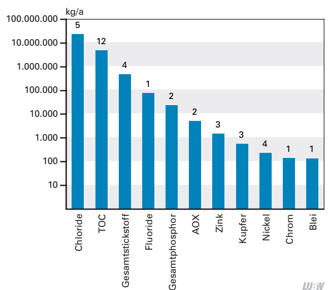
Abb. 6.5-3: Ins Gewässer freigesetzte Schadstofffrachten PRTR-pflichtiger Betriebe und jeweilige Anzahl der Betriebe im Jahr 2007 in Baden-Württemberg. Stand: 2008
