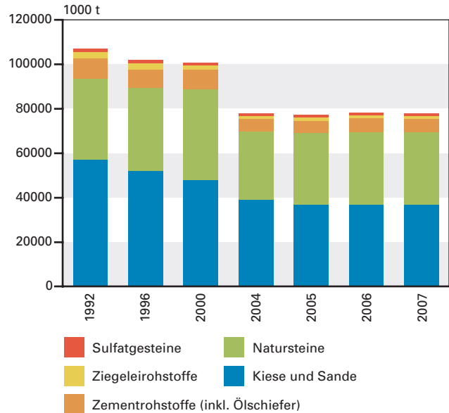
Abb. 2.1-2: Rohförderung mineralischer Rohstoffe. Nicht berücksichtigt: hochreine Kalksteine, Steinsalz/Sole, Fluss-/Schwerspat Quelle: Landesamt für Geologie, Rohstoffe und Bergbau Baden-Württemberg 2008
