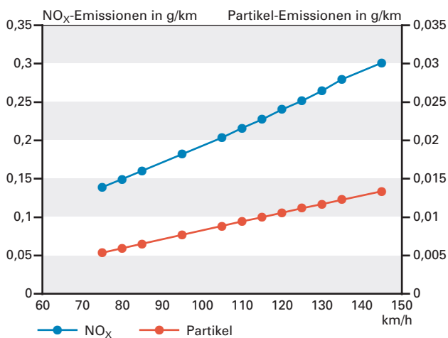
Abb. 4.2-5: Pkw-Emissionen auf Bundes-Autobahnen (BAB). Ausgewertet sind nur solche BAB-Verkehrssituationen, die eine konstante Geschwindigkeit aufweisen. Bezugsjahr 2008. [HBEFA 2004].
