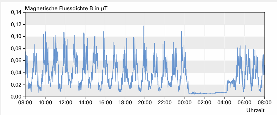
Tagesgang der magnetischen Flussdichte an der Ammergaubahn in Murnau am Staffelsee in ca. 80 m Entfernung von der Bahnstrecke.
