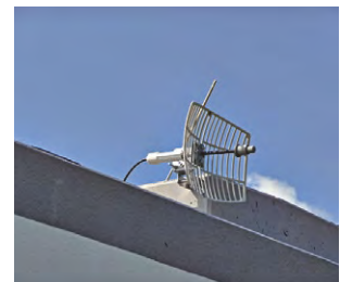
Abb. 70: WLAN-Richtfunksystem mit Gitter-Parabolantenne (5,8 GHz).
