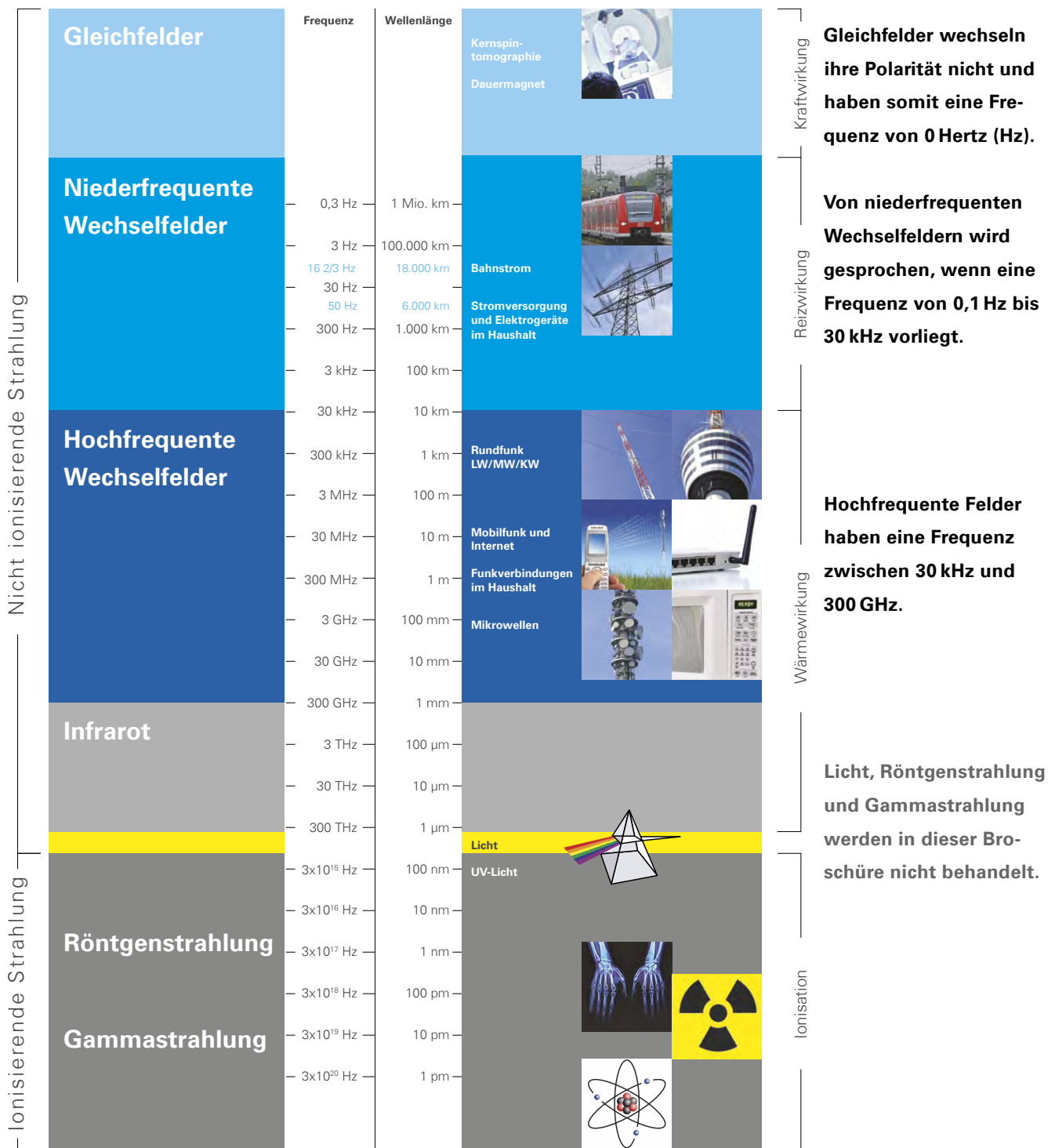
Abb. 8: Elektromagnetisches Spektrum
