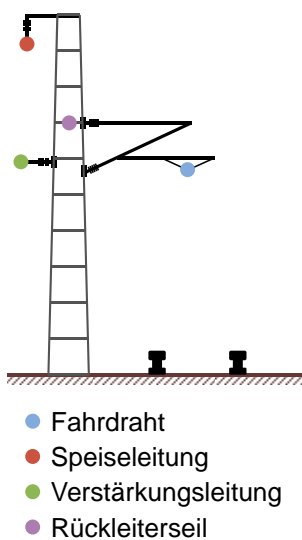
Abb. 29: Mögliche Leitungs-konfiguration auf einem Fahrleitungsmasten der DB.
